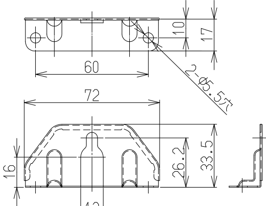
●取付金具上詳細図(S=1:2)
