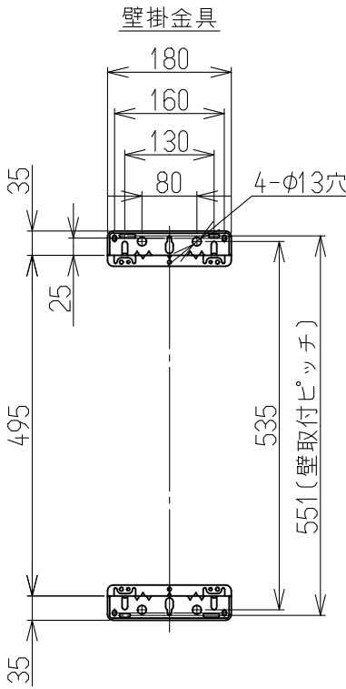
●取付金具下詳細図(S=1:2) 左右共通
