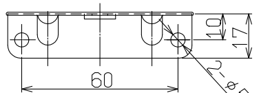
●取付金具上詳細図 (S=1:2)
