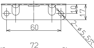
●取付金具上詳細図 (S=1:2)
