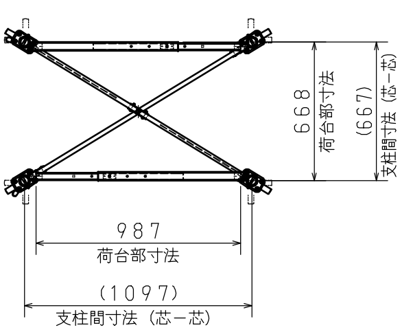
使用状態③ (S = 1 : 25)
