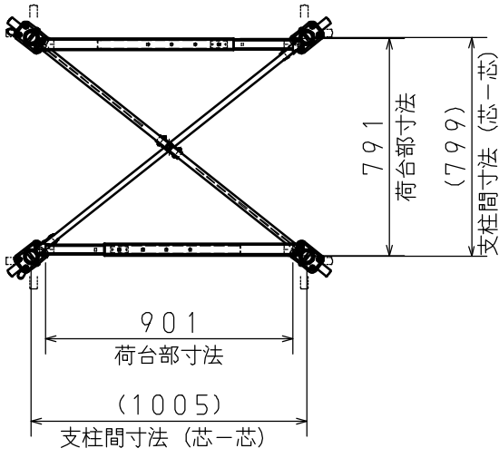
使用状態② (S = 1 : 25)
