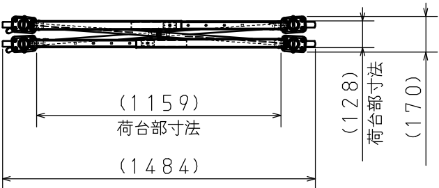
収納状態 (S = 1 : 25)
