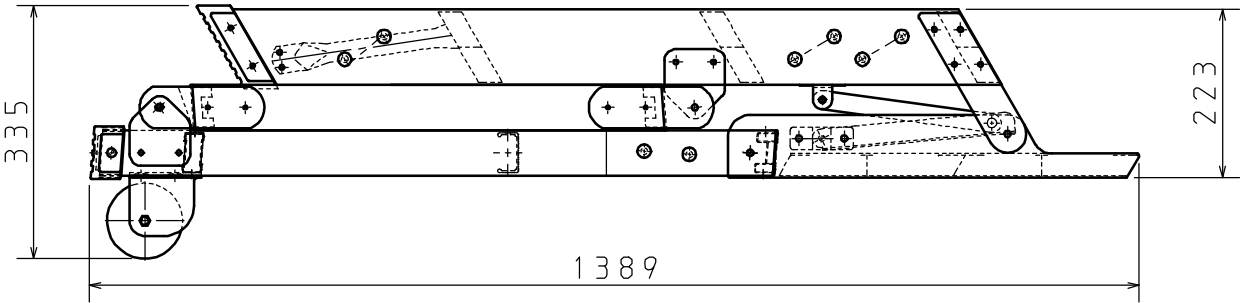
収納状態図
