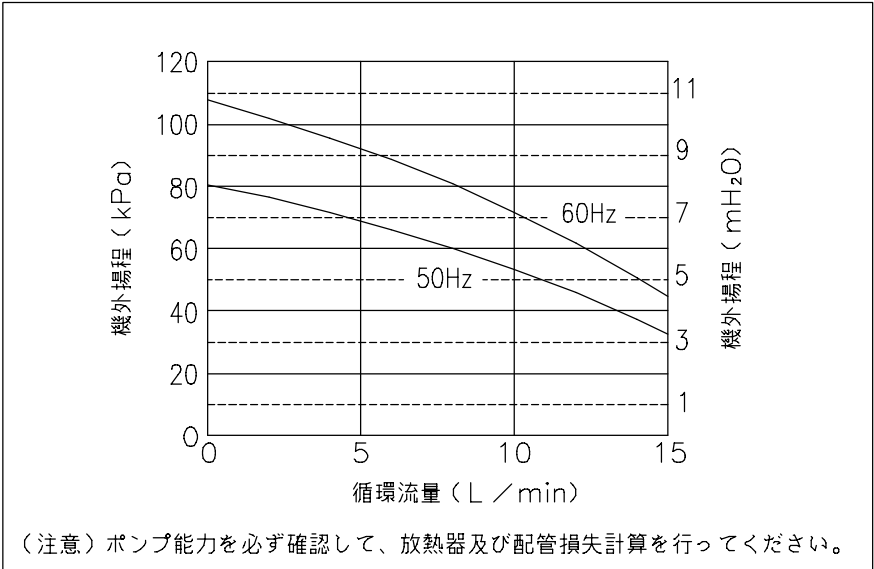
■ポンプ機外揚程
