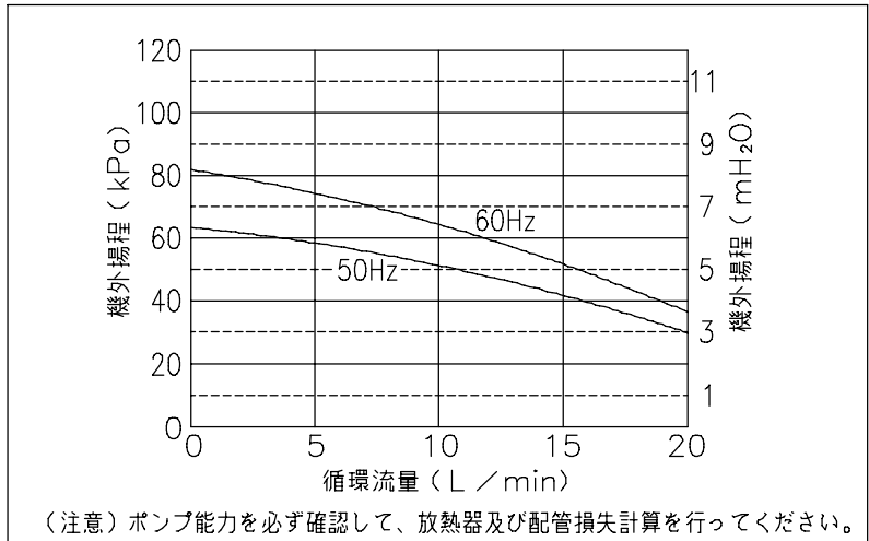
■ポンプ機外揚程
