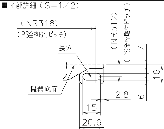
■イ部詳細（S=1/2）
