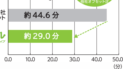
■研削スピード比較 (研削量400gまで)
