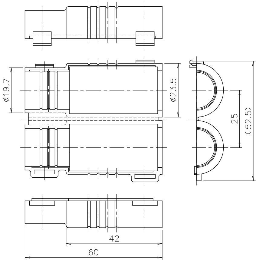
④ プロテクターキャップ 7A用 色：アイボリー 材質：軟質PP
