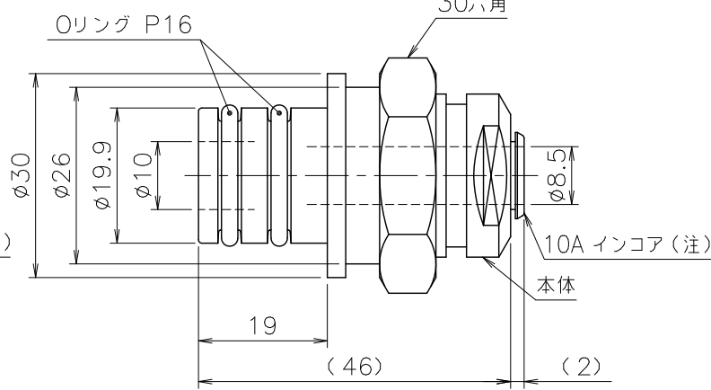
③ CHP2-10W MP (10Aインコア含む) 材質：黄銅 (C3604BD)
