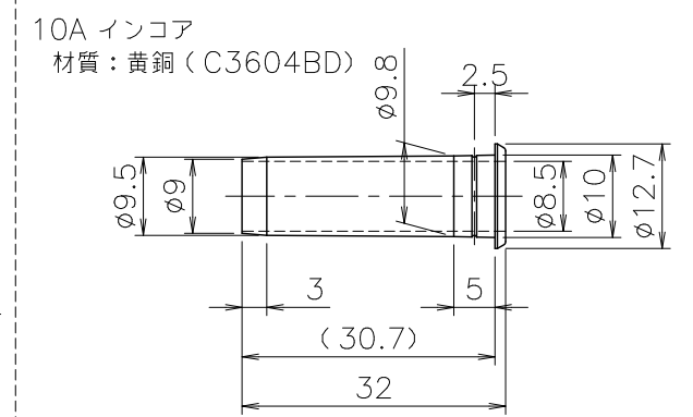
⑥ CHP1-10W (10Aインコア含む) 材質：黄銅 (C3604BD)
