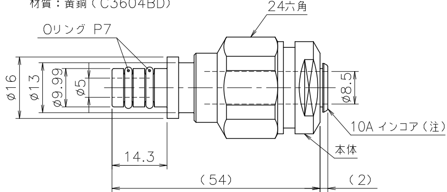
⑥ CHP1-10W (10Aインコア含む) 材質：黄銅 (C3604BD)
