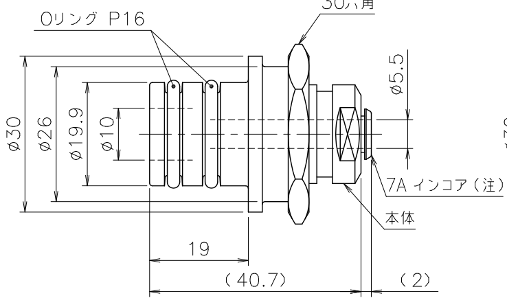
② CHP2-7W MP (7Aインコア含む) 材質：黄銅 (C3604BD)
