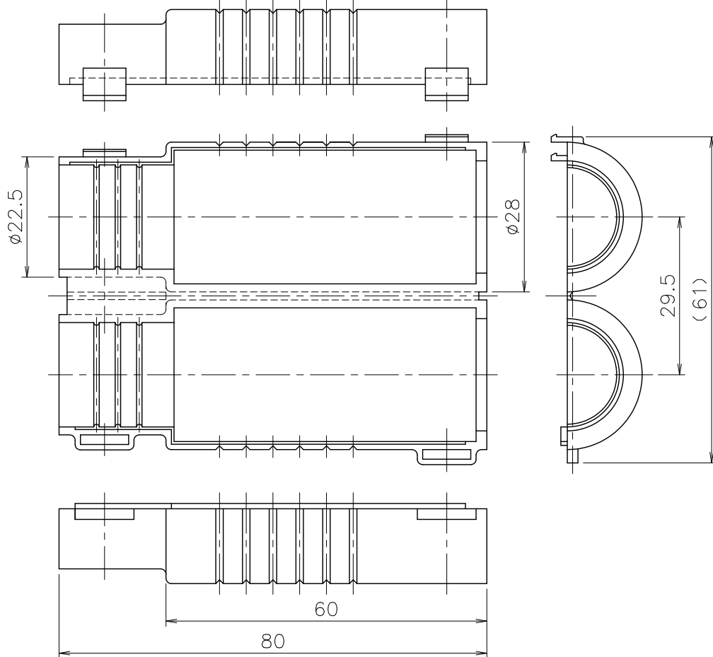
⑤ プロテクターキャップ 色：アイボリー 材質：軟質PP
