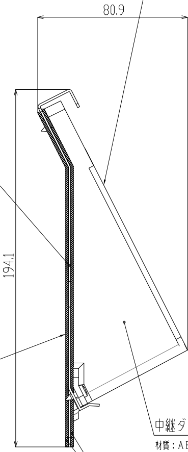
パッキン 材質：積水化学（株）製 ソフトロンS相当
