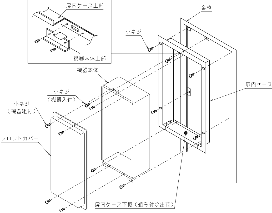
扉内ケース上部と機器本体上部の取付要領図
