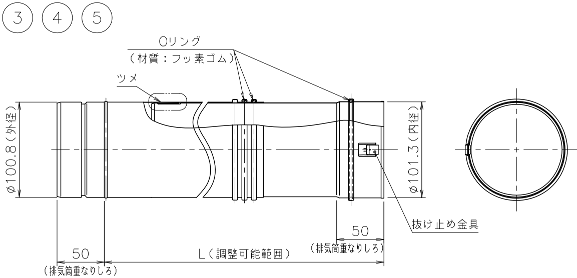
■寸法表
