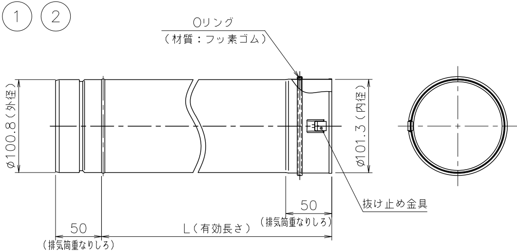
■寸法表
