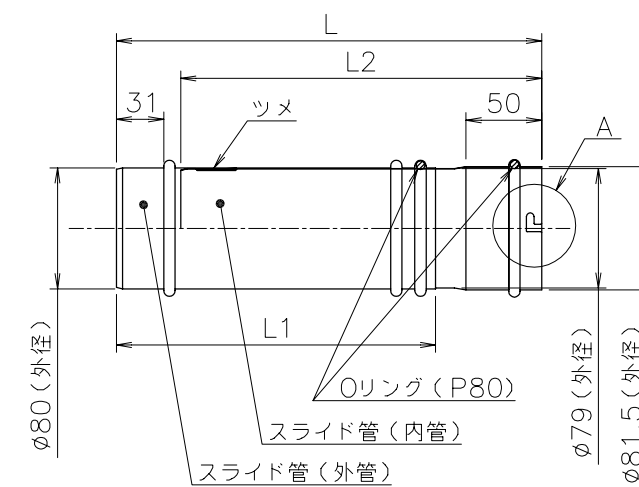
■ 寸法表
