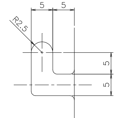
■A部詳細図（尺度 2：1）
