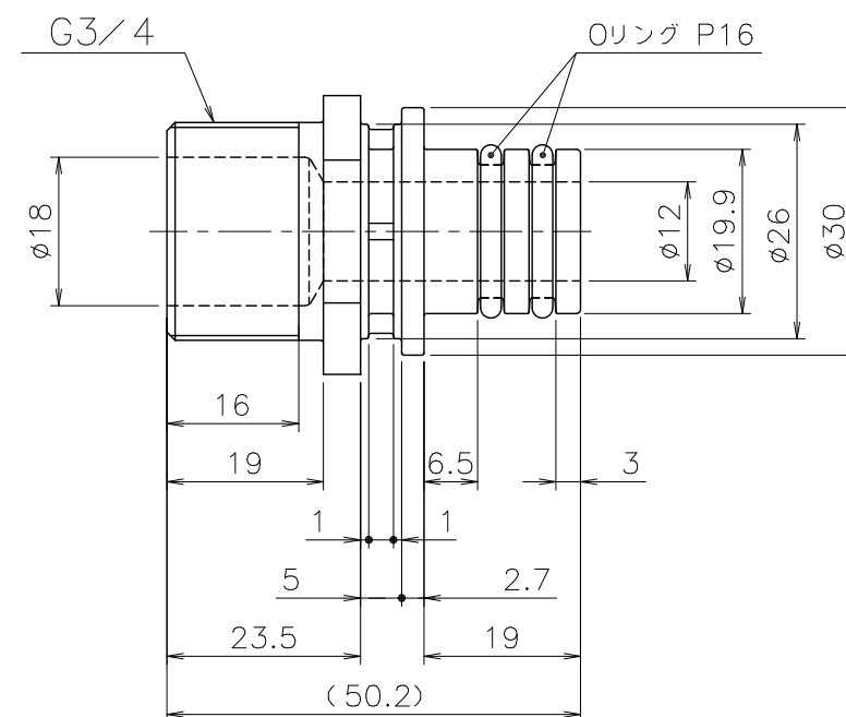
② CHP2-MP20J×1 材質：PPS
