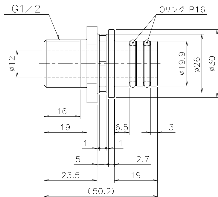
① CHP2-MP15J×1 材質：PPS
