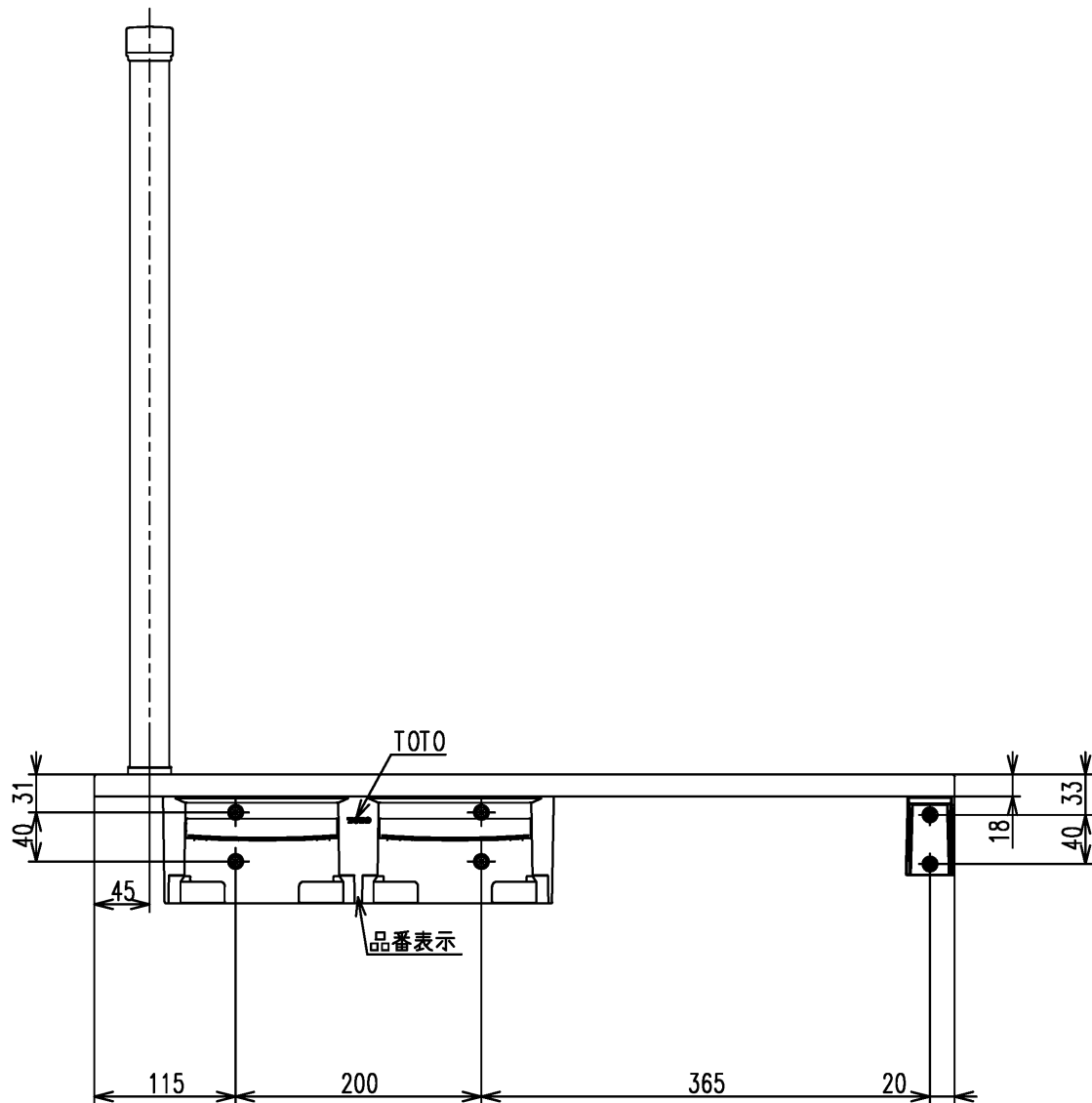
左壁設置の場合
