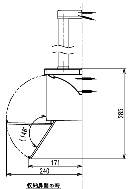
右壁設置の場合(1:10)
