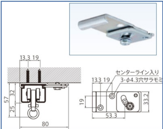
レール断面図 単位:mm
