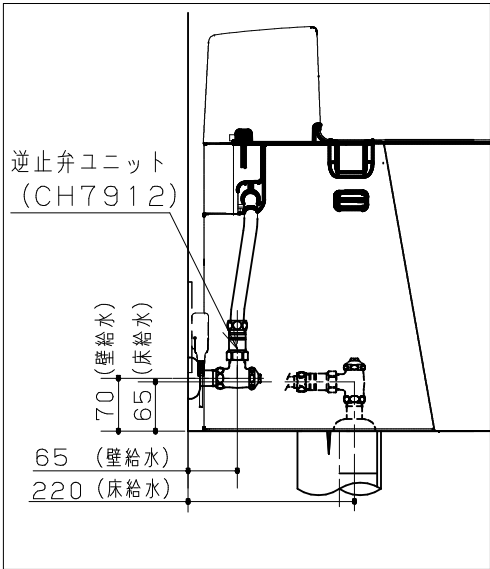
逆止弁ユニット (CH7912) 使用の場合の給水位置
