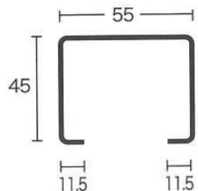
・上からの支柱断面図
