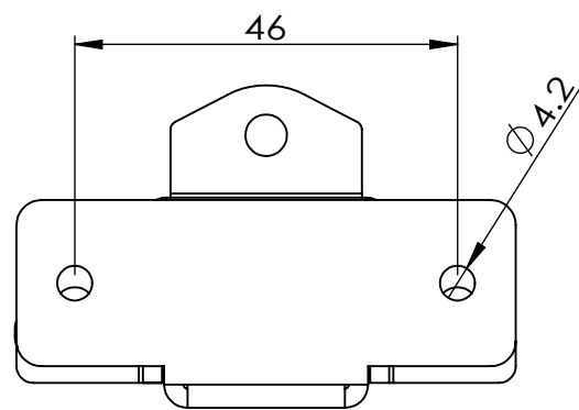
矢視図 A-A
