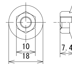
皿ばねナット詳細図
