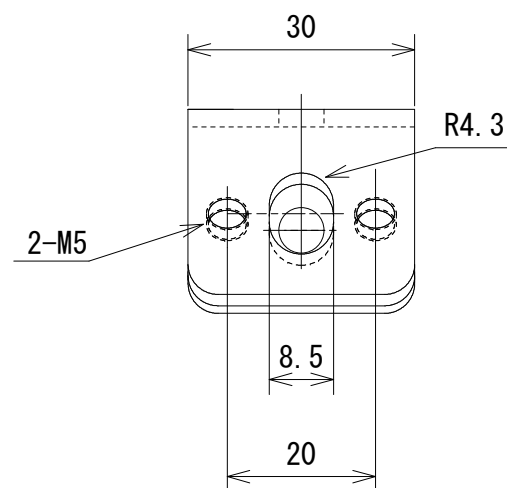
〈正面図〉
