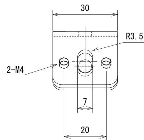
〈正面図〉
