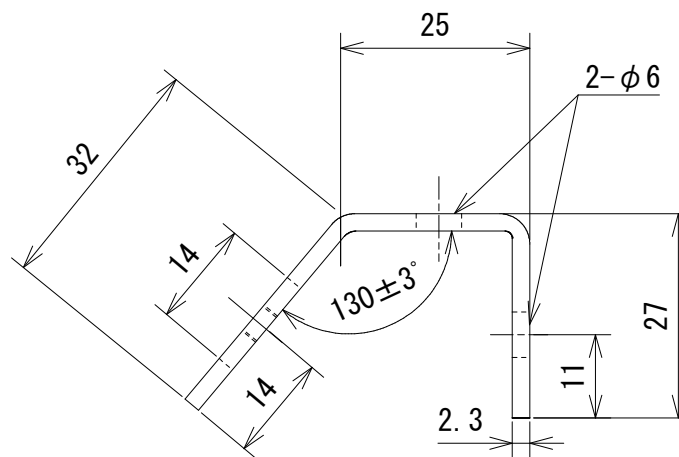
〈側面図〉
