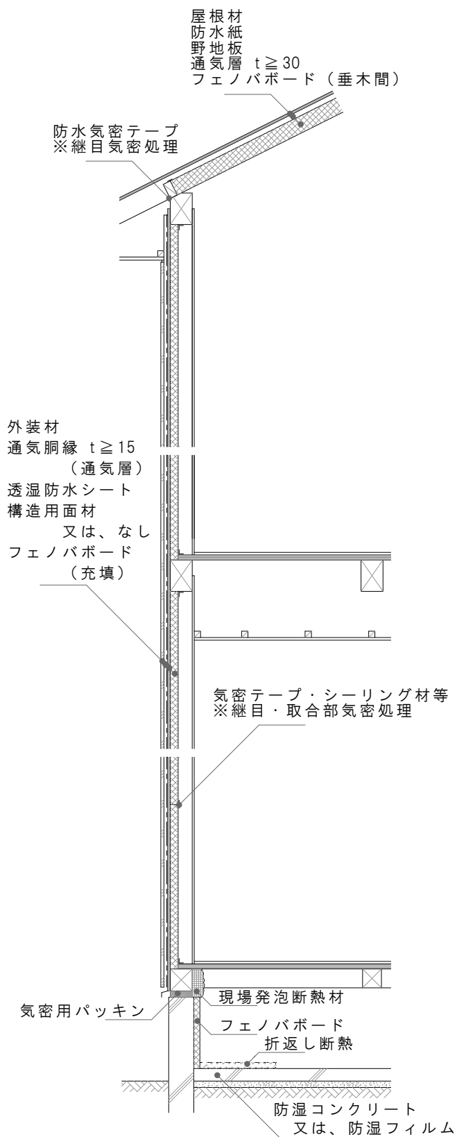
屋根・基礎断熱
