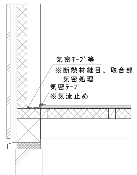
(ii) 根太直行断面
