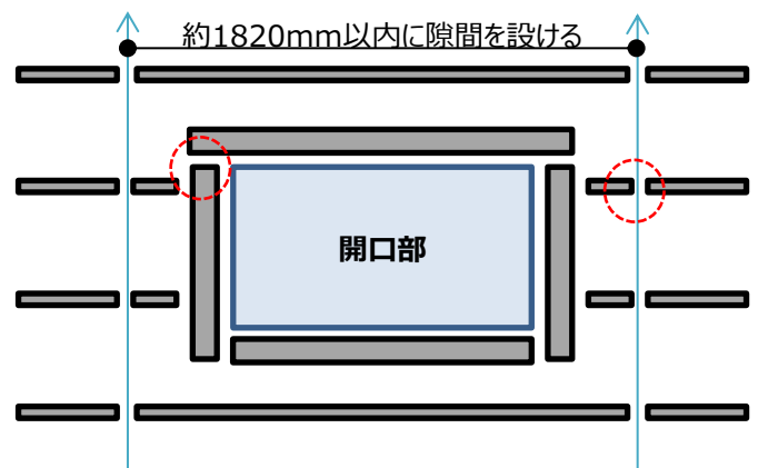
横胴縁の場合
