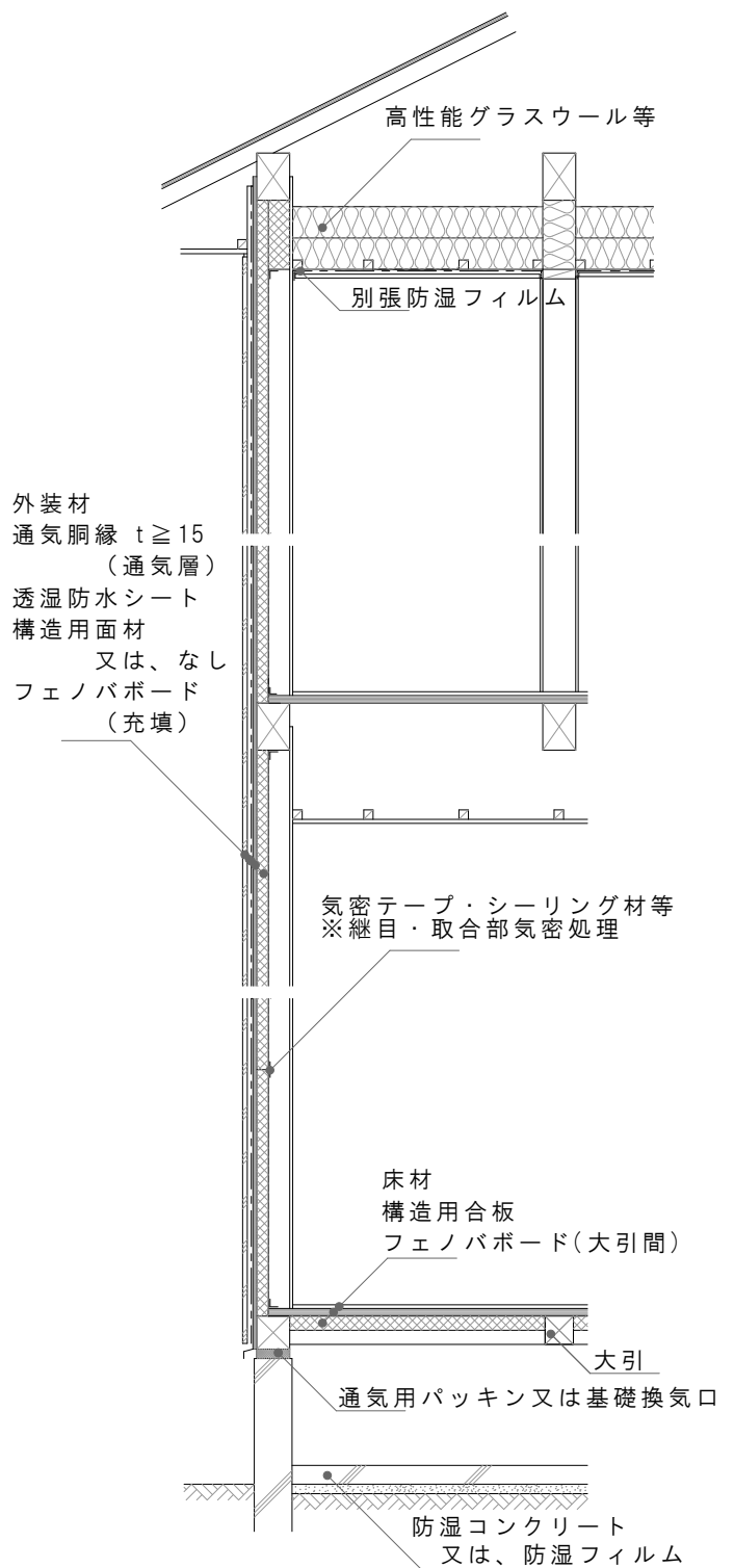
天井・床断熱
