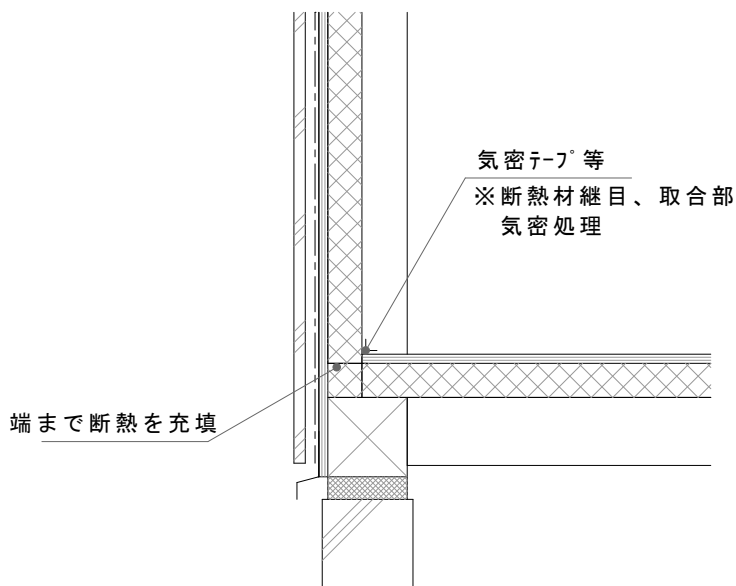
(i) 根太平行断面
