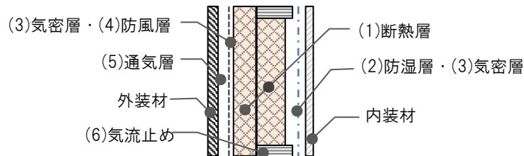
付加断熱工法の層構成の一例
