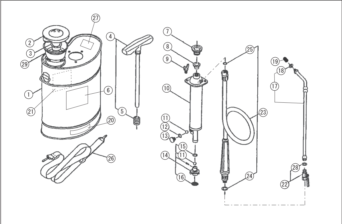
型式名 SS-4DX-AAA-1 (042850403)
