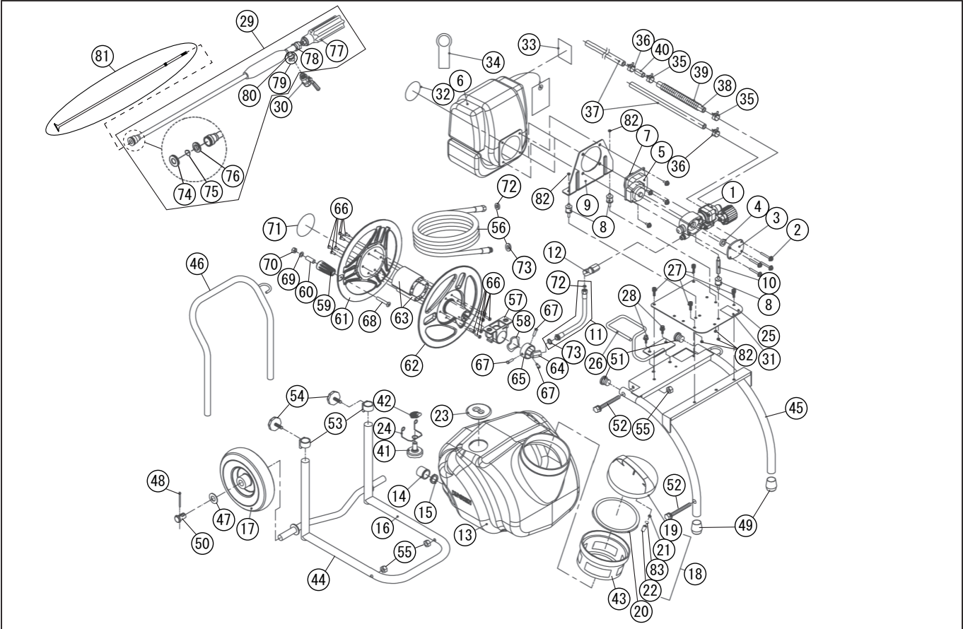
型式名 ES-25T-AAA-0 <KC26> (045878212)
