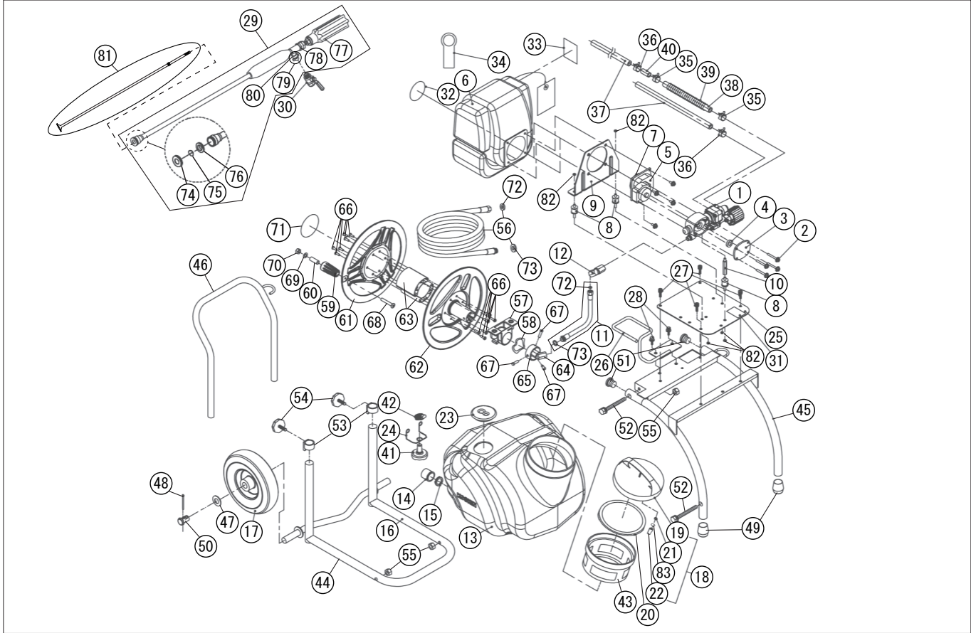
型式名 ES-25T-AAA-0〈KC26〉(045891506) 減速機クミ
