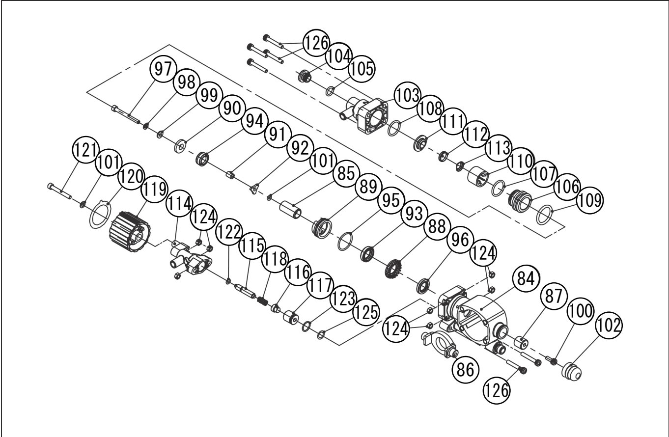
型式名 ES-25T-AAA-0 〈KC26〉 (045878212) ポンプクミ
