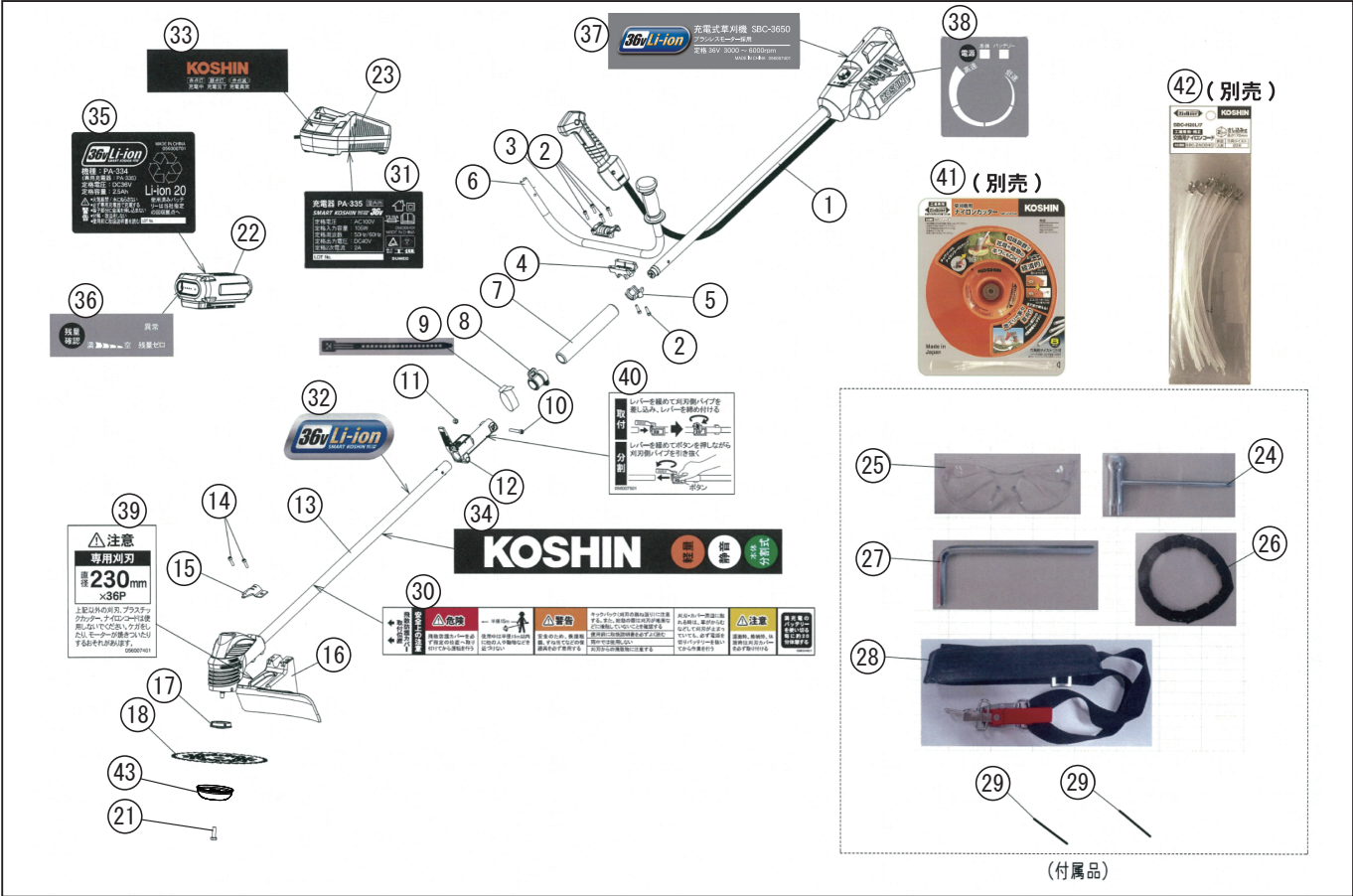
型式名 SBC-3650-AAA-1 (056855103)
