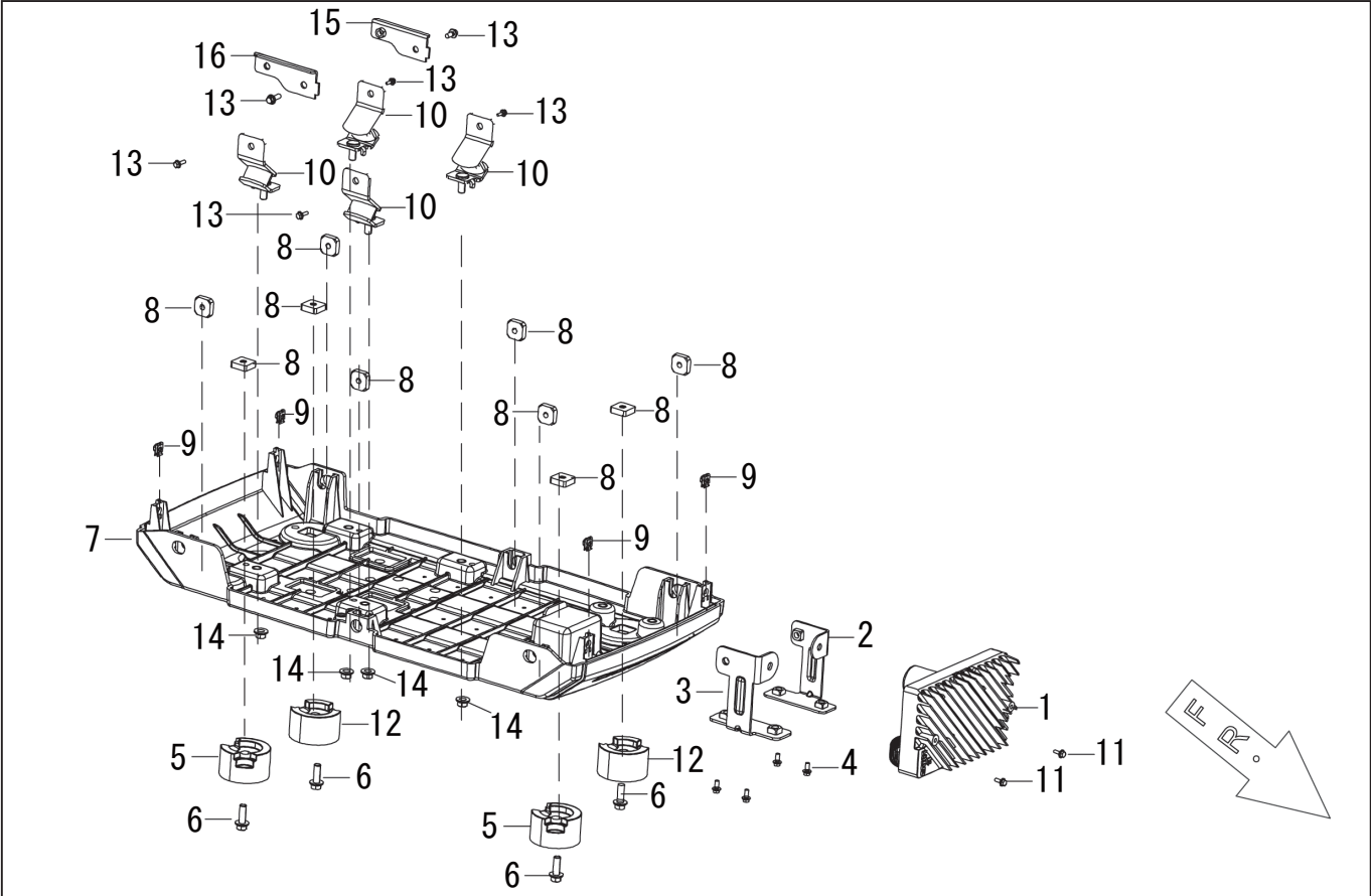
型式名 GV-16SE-AAA-0 (065864601) インバーター、底板
