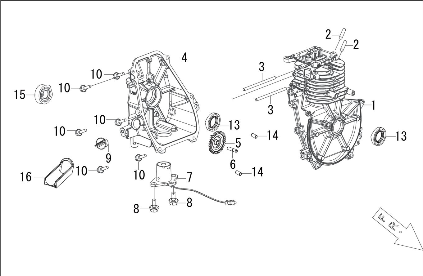
型式名 GV-16SE-AAA-0 (065864601) クランクケース、ケースカバー
