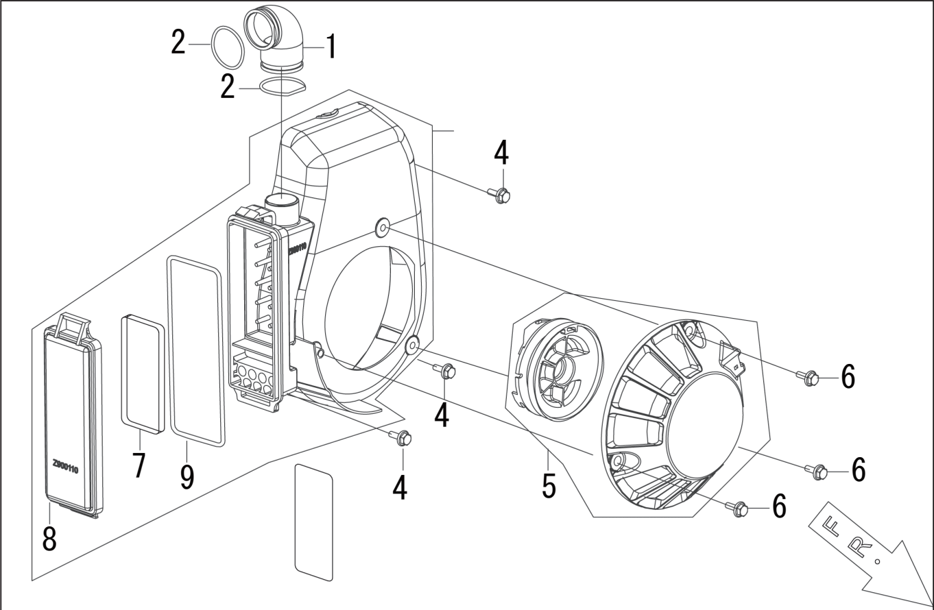
型式名 GV-16SE-AAA-0 (065864601) ファンカバー、リコイルスターター
