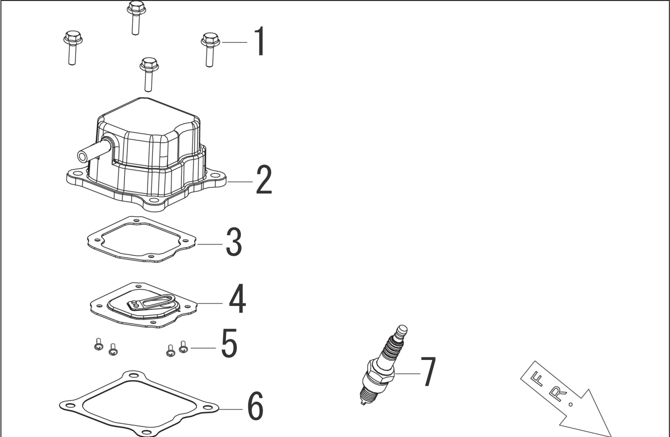
型式名 GV-16SE-AAA-0 (065864601) シリンダーヘッド、スパークプラグ
