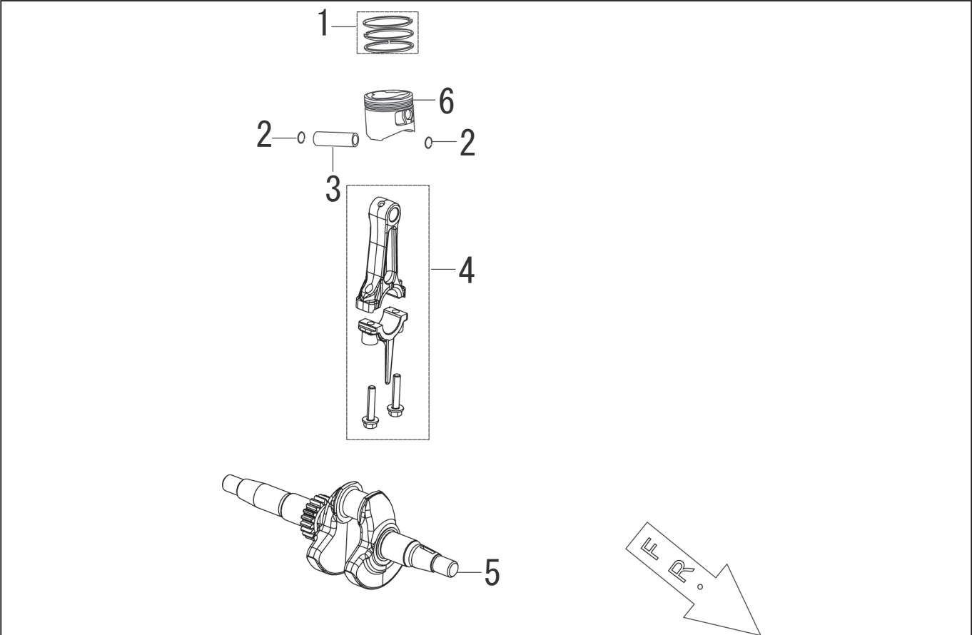
型式名 GV-16SE-AAA-0 (065864601) ピストン、クランクシャフト
