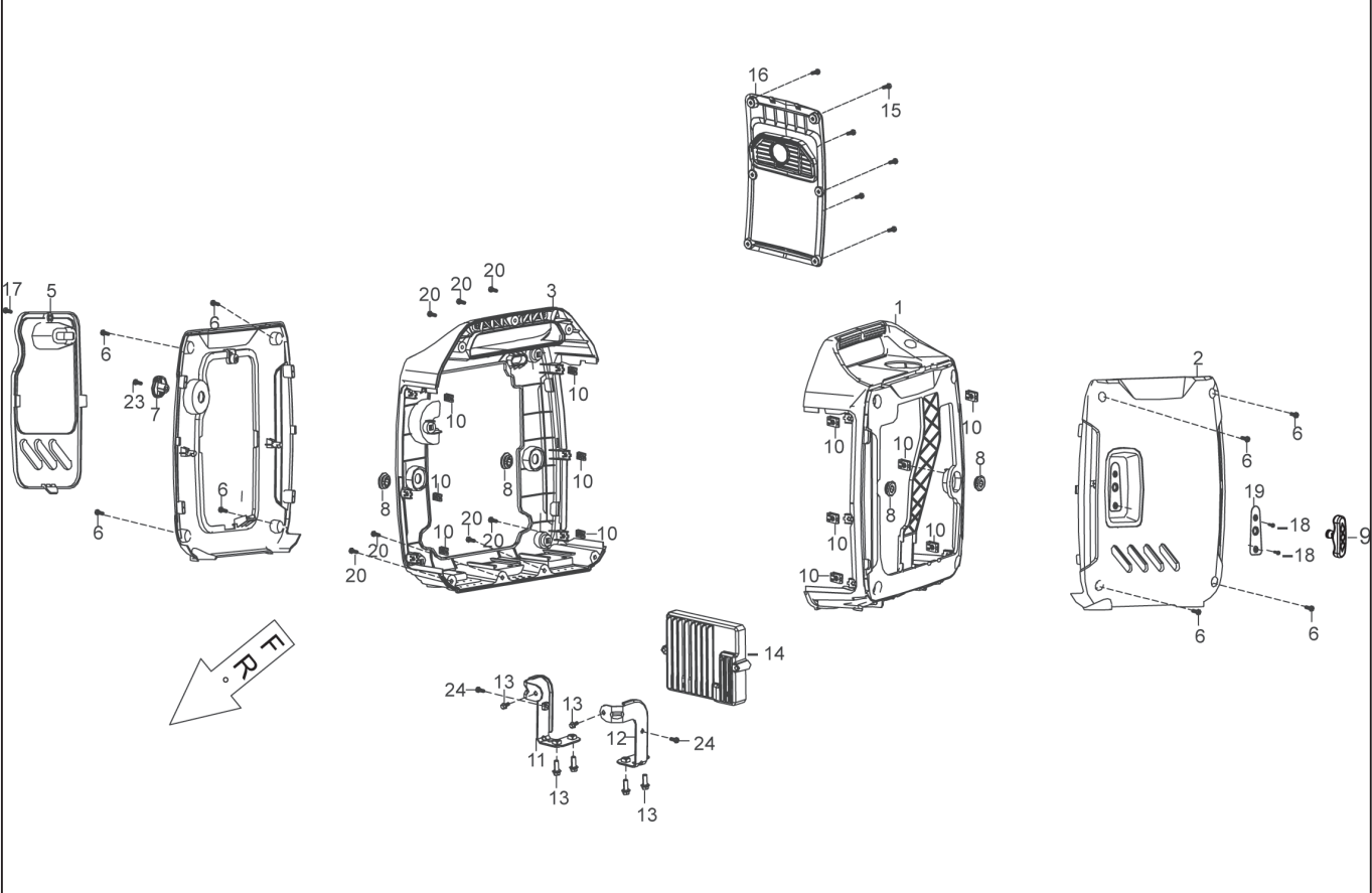
型式名 GV-9SE-AAA-0 (065864501) カバー
