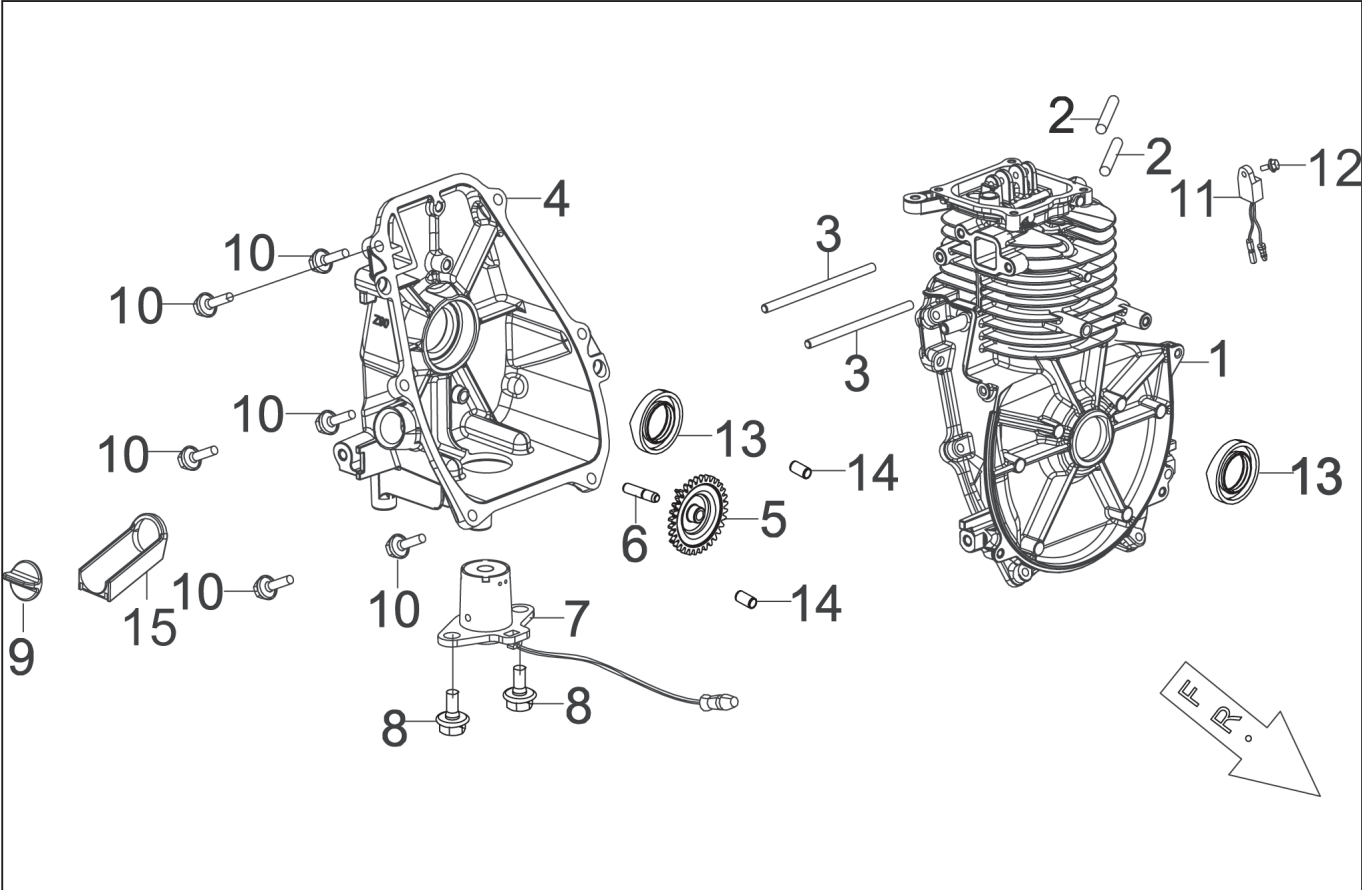
型式名 GV-9SE-AAA-0 (065864501) クランクケース、ケースカバー
