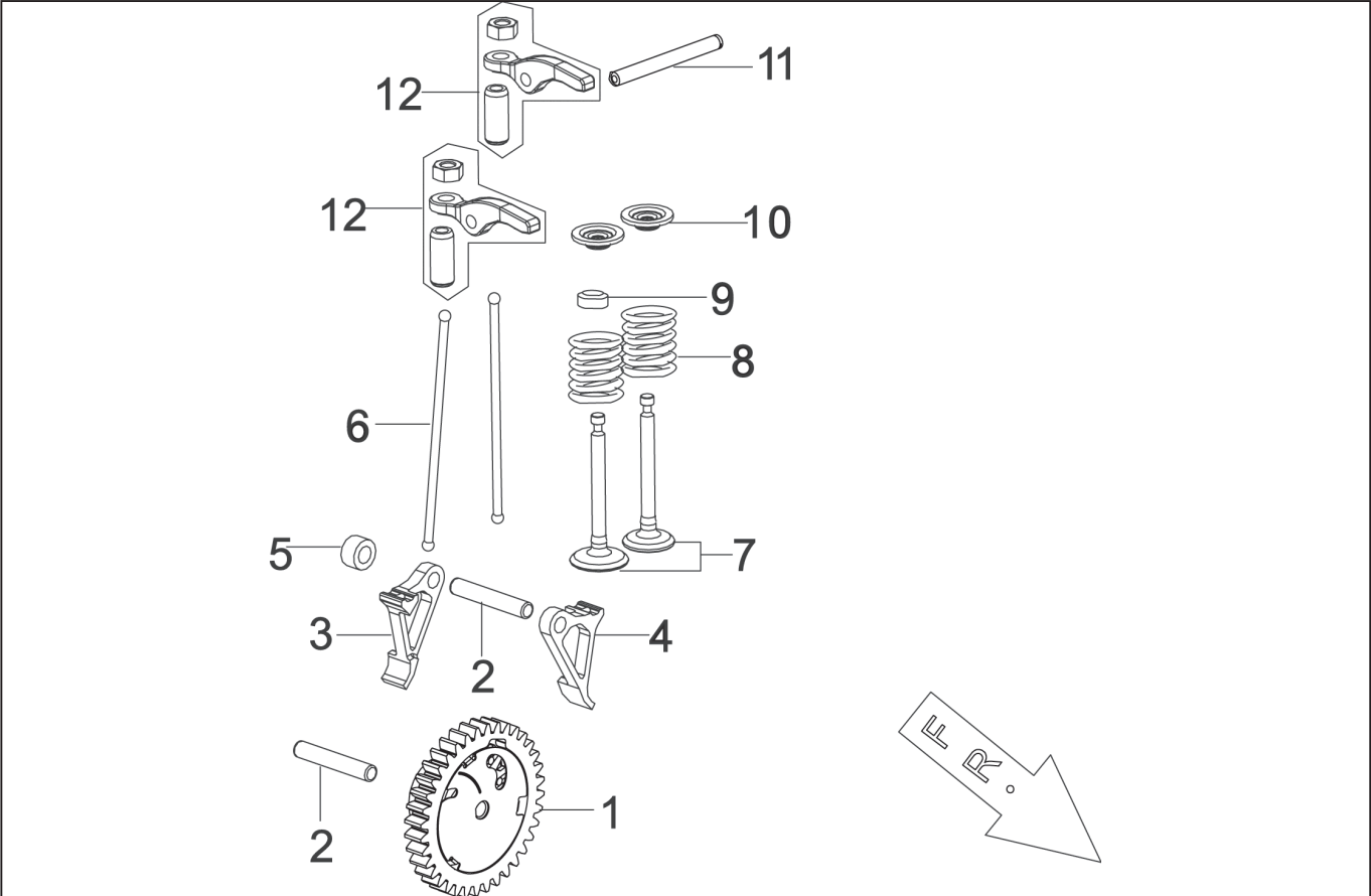
型式名 GV-9SE-AAA-0 (065864501) バルブ、カムシャフト
