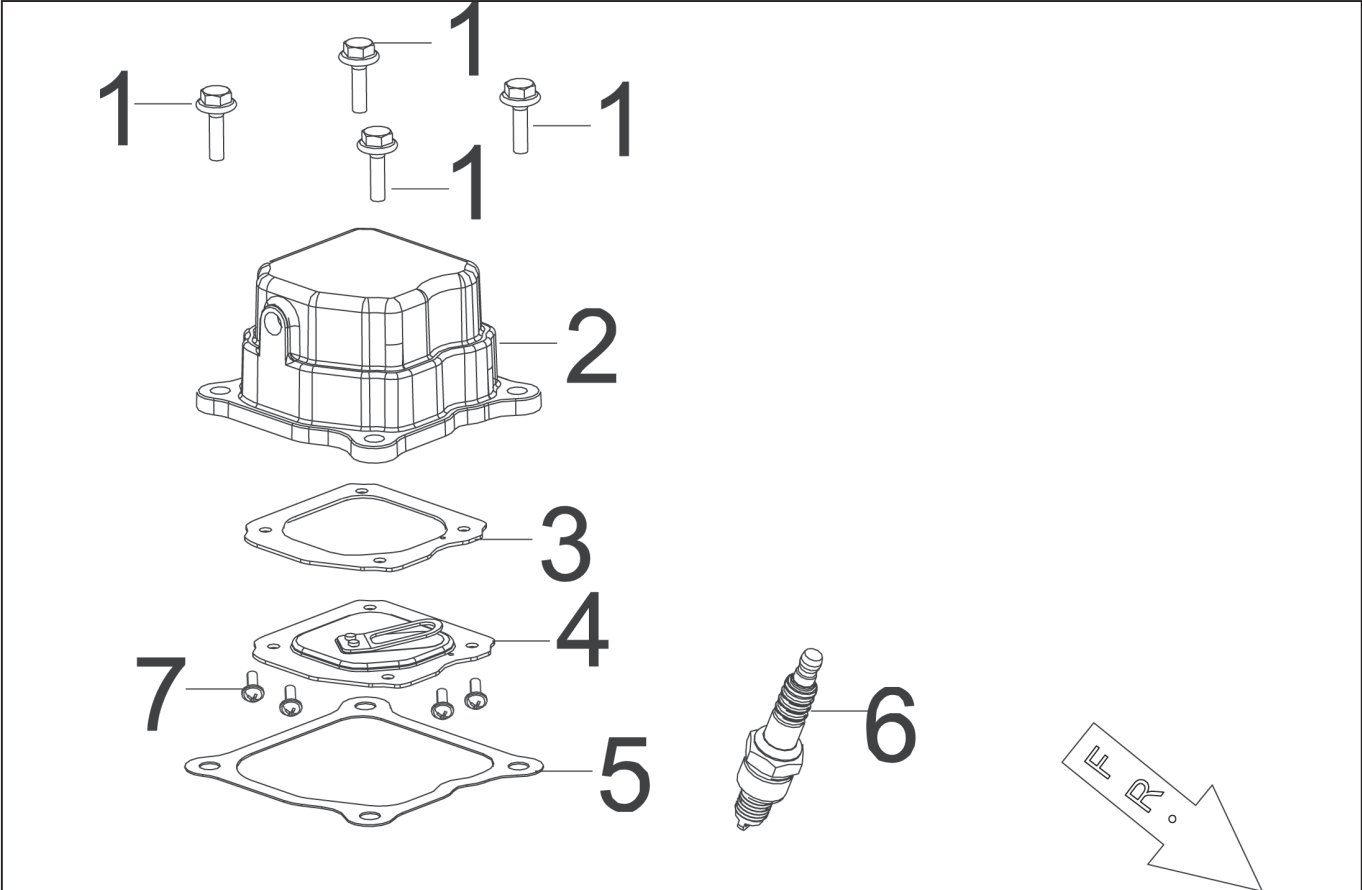
型式名 GV-9SE-AAA-0 (065864501) シリンダーヘッド、スパークプラグ
