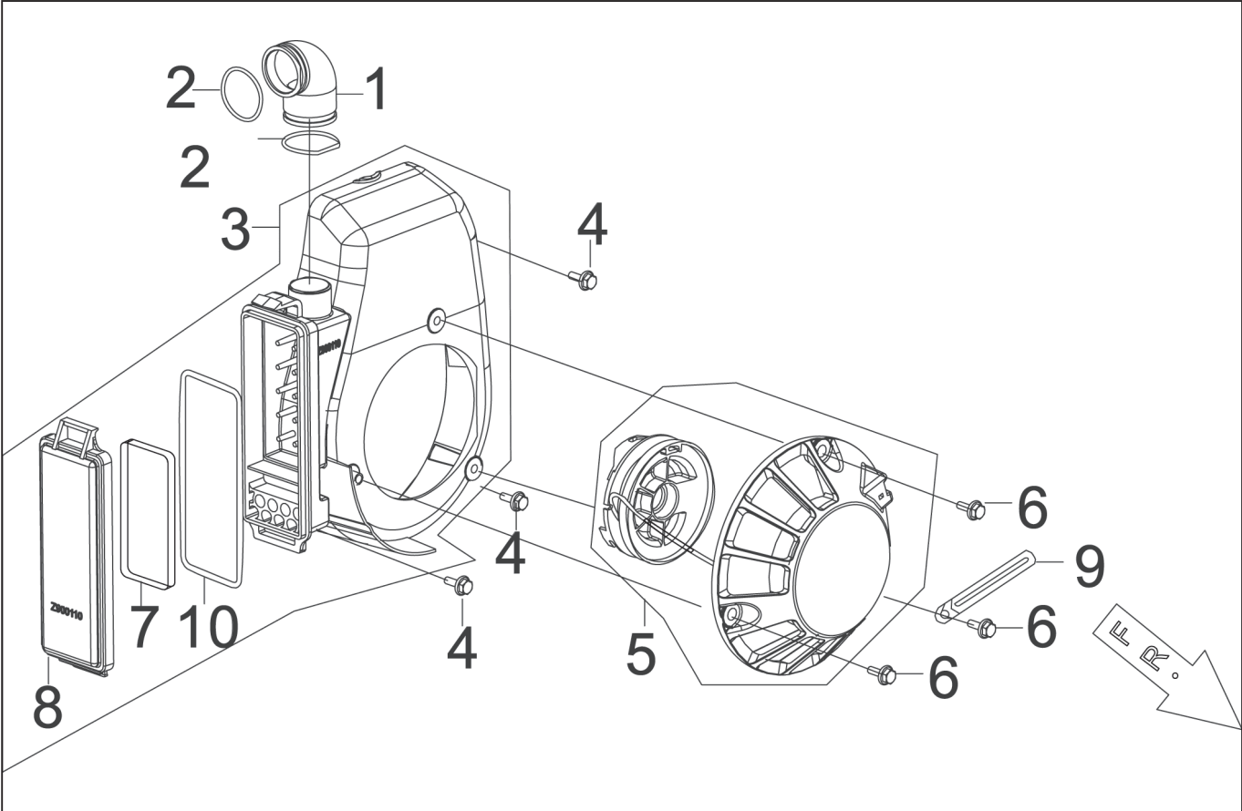
型式名 GV-9SE-AAA-0 (065864501) ファンカバー、リコイルスターター
