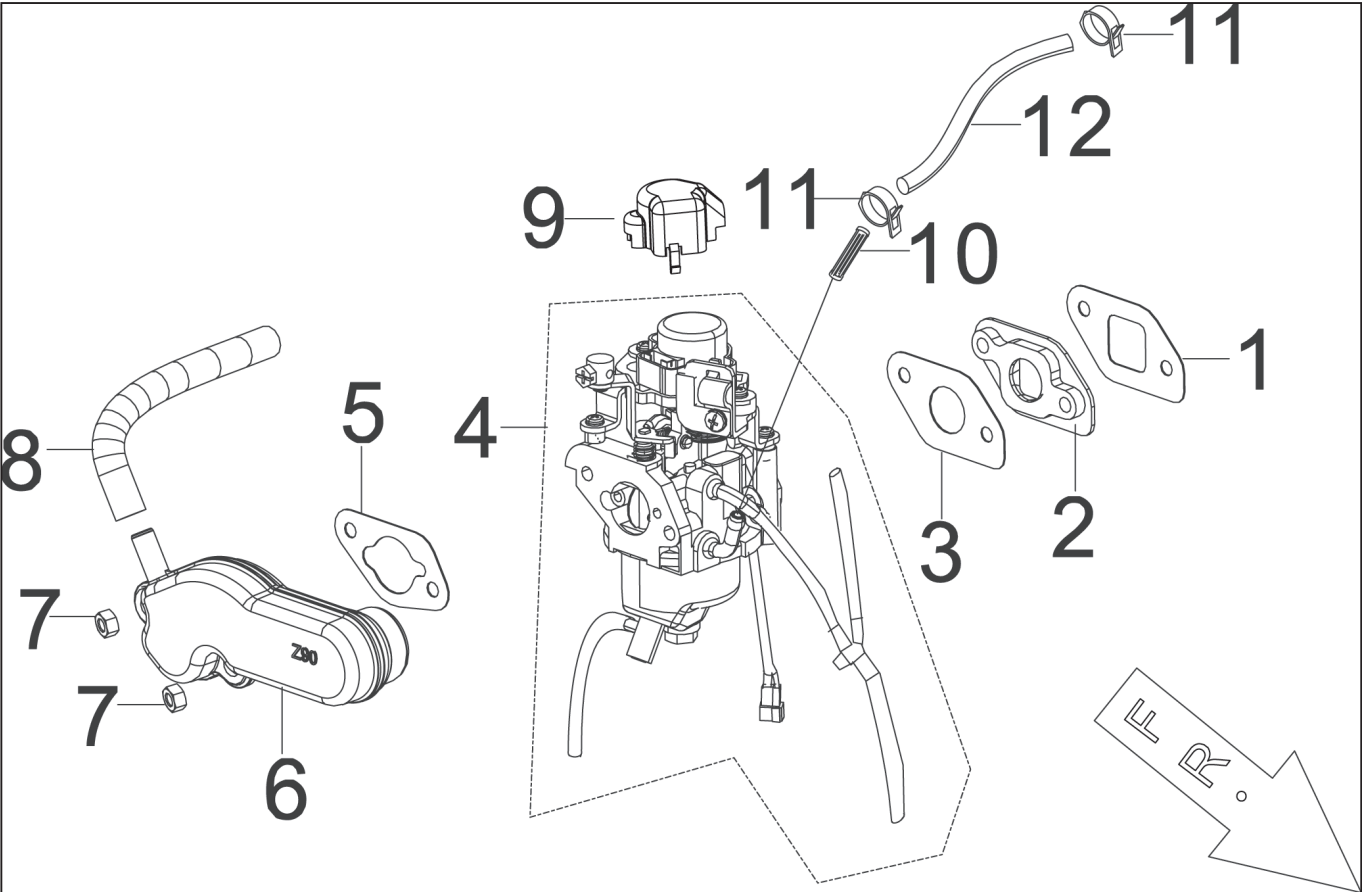
型式名 GV-9SE-AAA-0 (065864501) キャブレター
