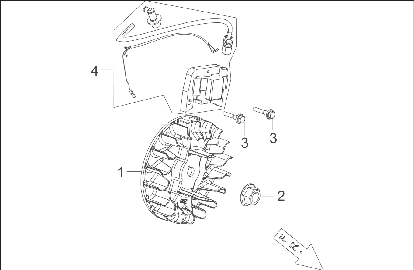
型式名 GV-9IG-AAA-0 (065864401) フライホイール、イグニッションコイル
