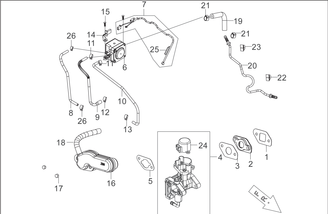
型式名 GV-9IG-AAA-0 (065864401) キャブレター
