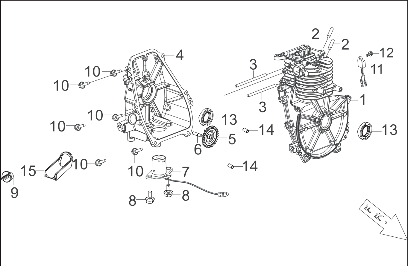
型式名 GV-9IG-AAA-0 (065864401) クランクケース、ケースカバー
