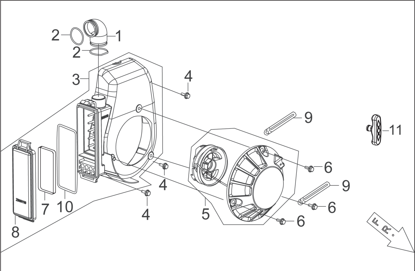
型式名 GV-9IG-AAA-0 (065864401) ファンカバー、リコイルスターター
