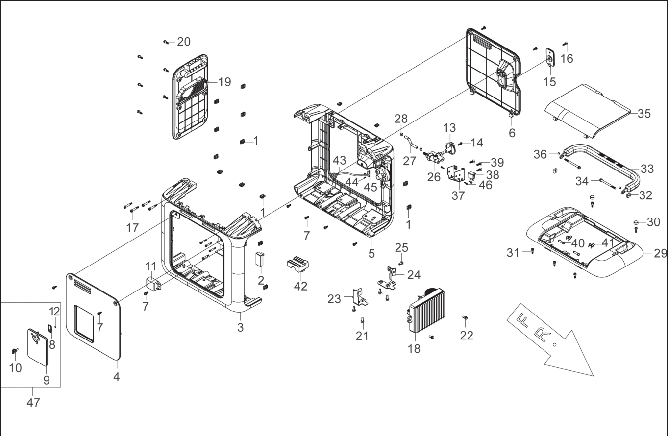
型式名 GV-9IG-AAA-0 (065864401) カバー
