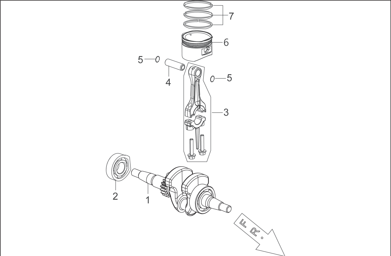
型式名 GV-9IG-AAA-0 (065864401) ピストン、クランクシャフト
