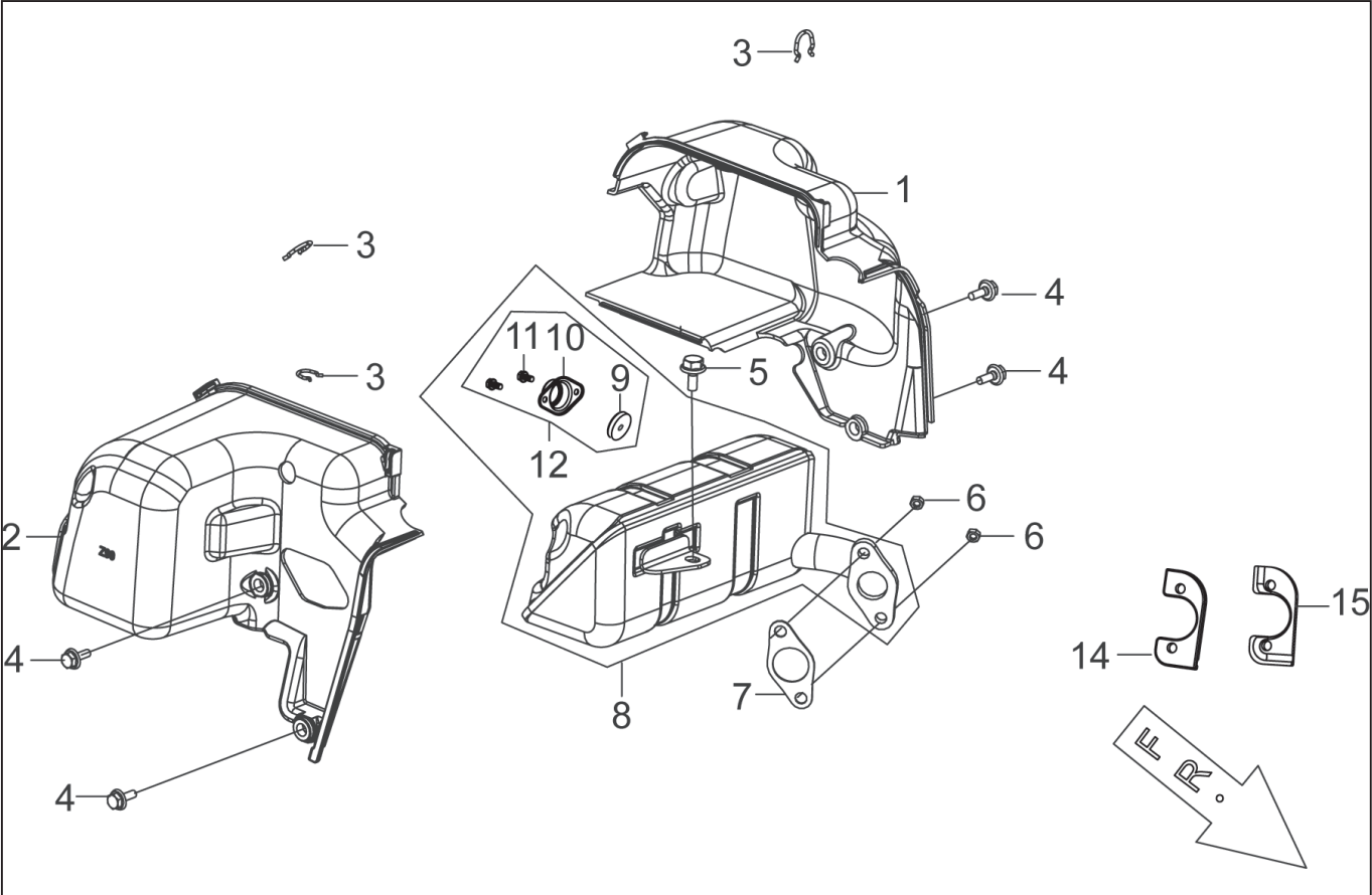
型式名 GV-9IG-AAA-0 (065864401) マフラー
