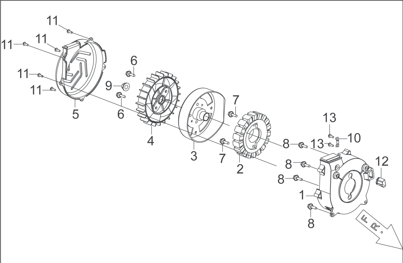
型式名 GV-9IG-AAA-0 (065864401) ローター、ステーター
