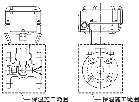
図9 保温施工
