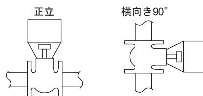
図7 取付姿勢（良い例）
