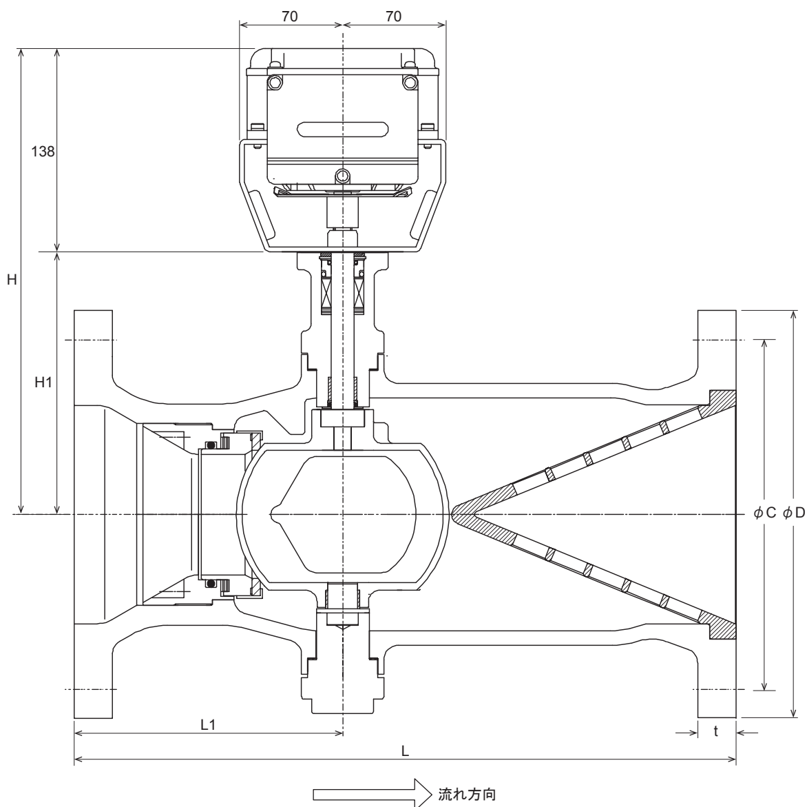
図4 外形寸法（接続口径 100A～150A 正面）（mm）
