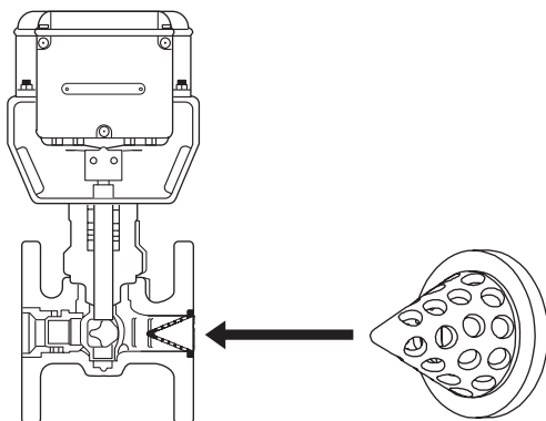
図1 耐キャビテーションエロージョン機構の構造
