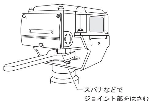
図11 手動開閉操作
