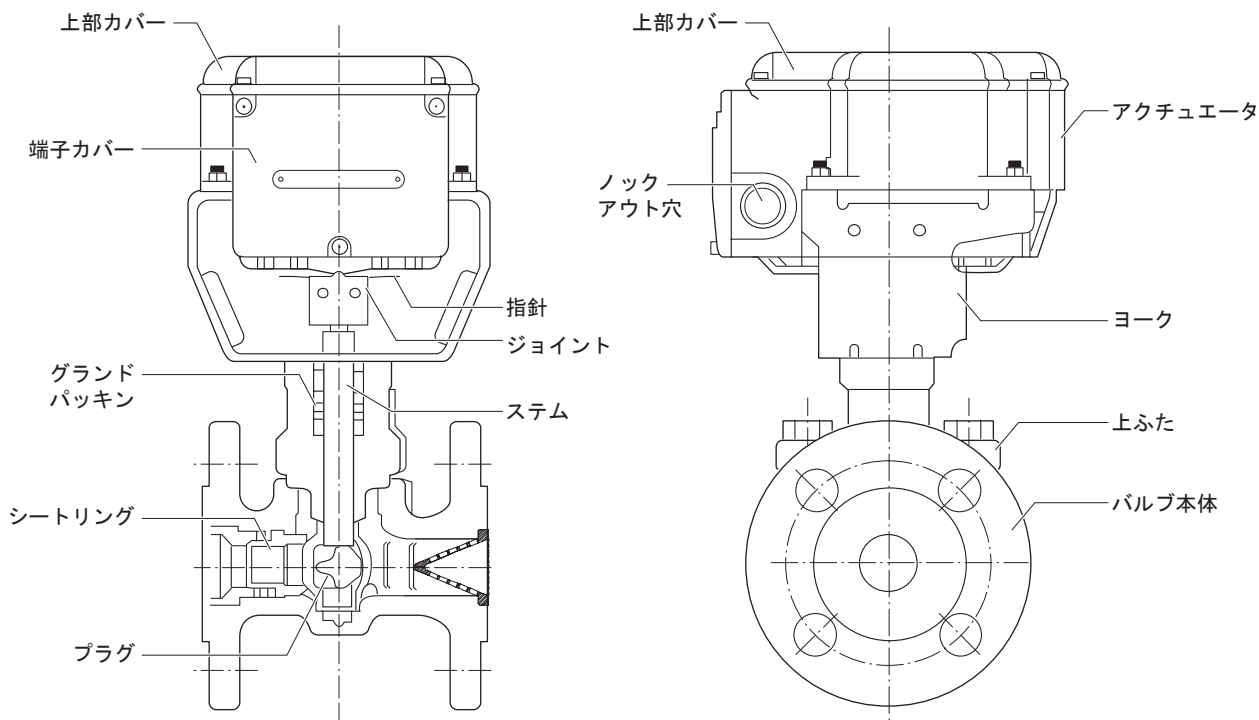
図6 各部の名称
