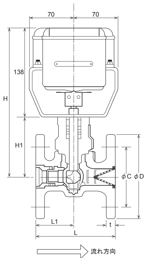
図2 外形寸法図（接続口径 15A～80A 正面）（mm）
