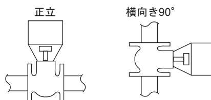
図4 取付姿勢（良い例）
