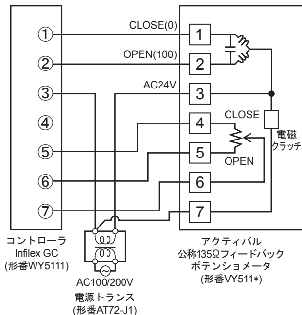
図 13 Inflex GC との接続例
