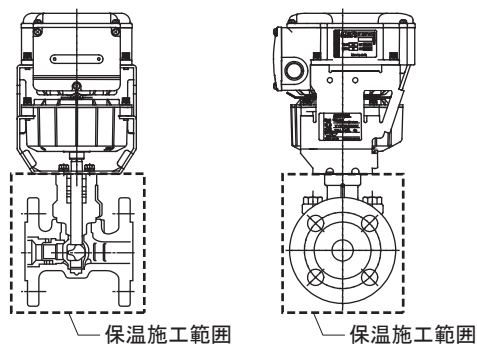
図6 保温施工
