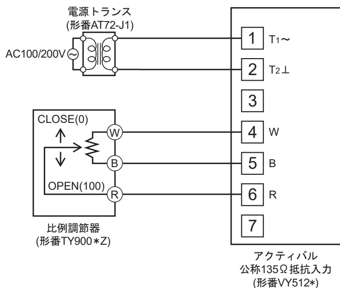
図 14 ネオスタートとの接続例
