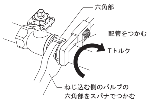
図7 配管への取り付け
