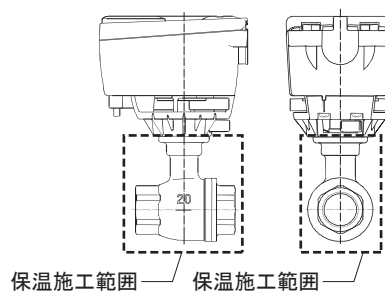
図8 保温施工 (15A~25A)
