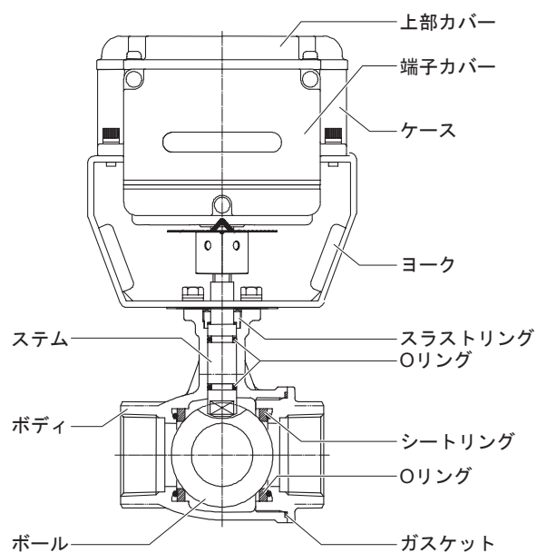
図4 接続口径32A（形番VY6300*2031）、接続口径40A（形番VY6300*2041）、接続口径50A（形番VY6300*2051）内部構造図
