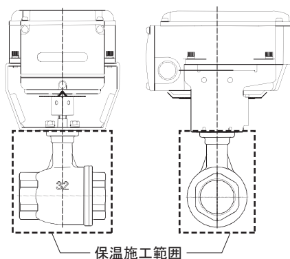
図11 保温施工 (32A~50A)
