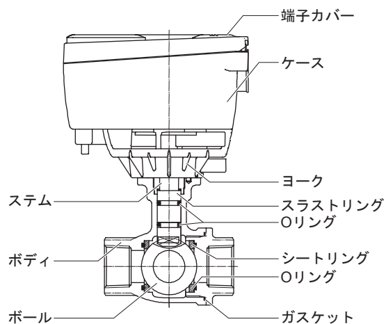
図3 接続口径15A（形番VY6300*2011）、接続口径20A（形番VY6300*2021）、接続口径25A（形番VY6300*2022）内部構造図
