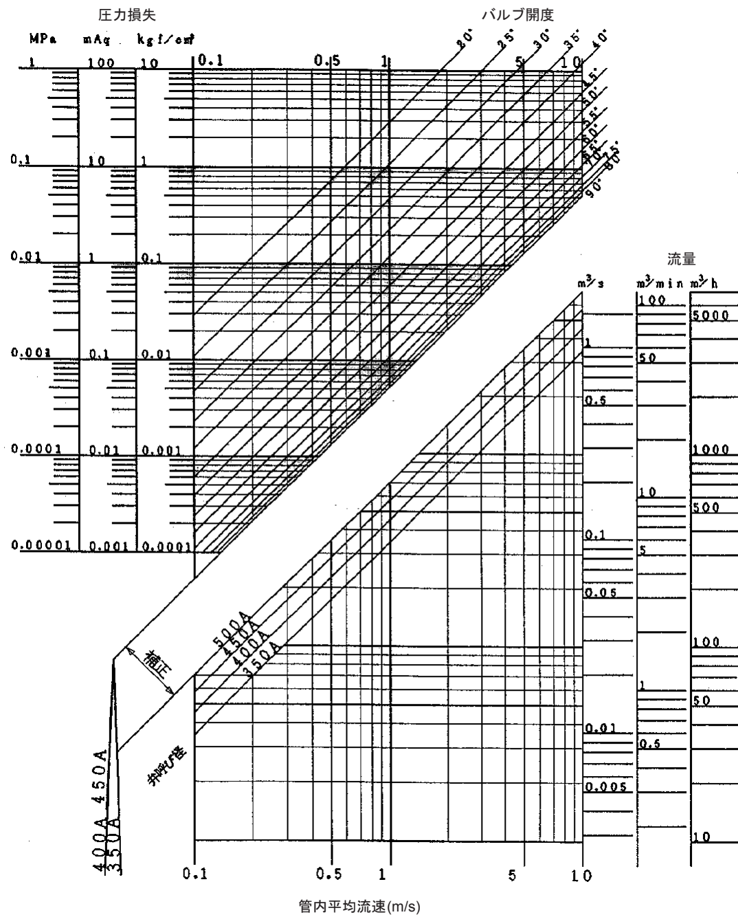
図34 形番VY6972、形番VY9972/バルブ接続口径選定および圧力損失線図 (バルブ接続口径350~500A、流体:水)
