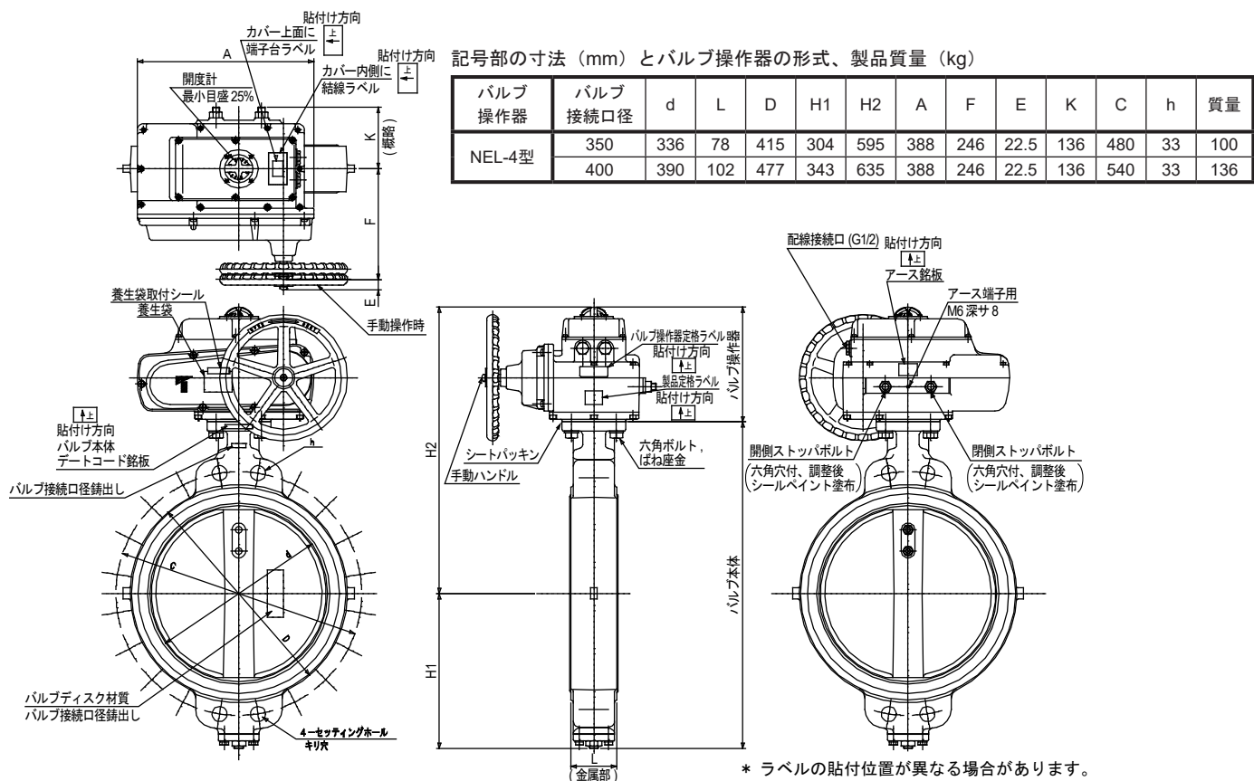
図14 形番VY6972（スピコンあり）バルブ接続口径350～400Aの形状・寸法 （図の形状はバルブ接続口径 400A、全閉状態の場合）
