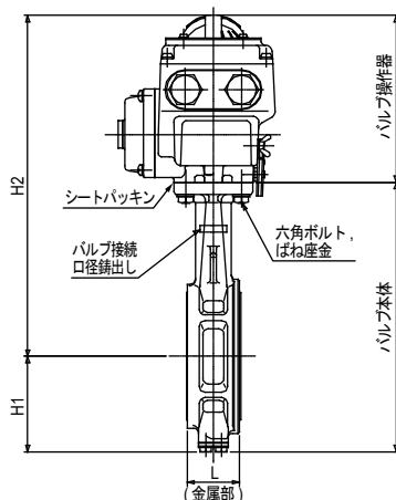
図9 形番VY6972、形番VY9972バルブ接続口径50～80Aの形状・寸法
