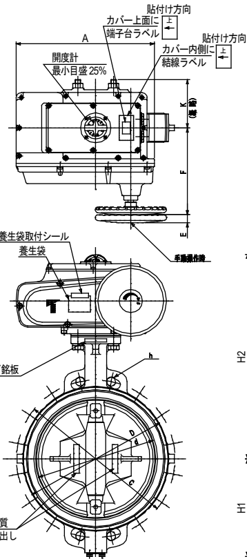
記号部の寸法 (mm) とバルブ操作器の形式、製品質量 (kg)
