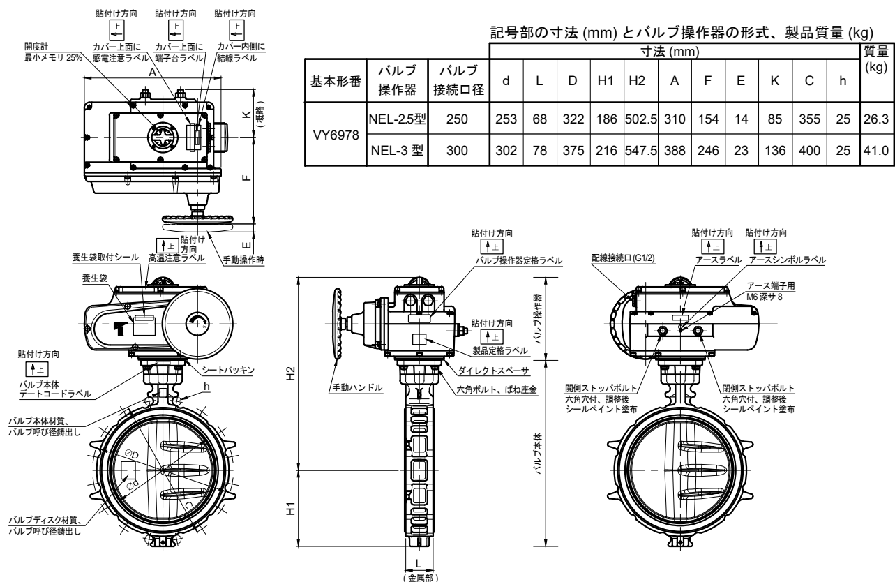
図18 形番VY6978バルブ接続口径250～300Aの形状・寸法 (図の形状はバルブ接続口径300A、全閉状態の場合)
