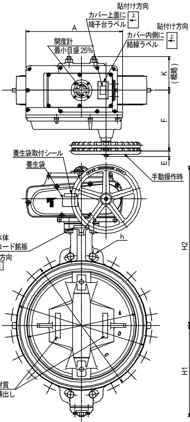
図6 形番VY6971（スピコンなし）バルブ接続口径450～500Aの形状・寸法 (図の形状はバルブ接続口径 450A、全閉状態の場合)
