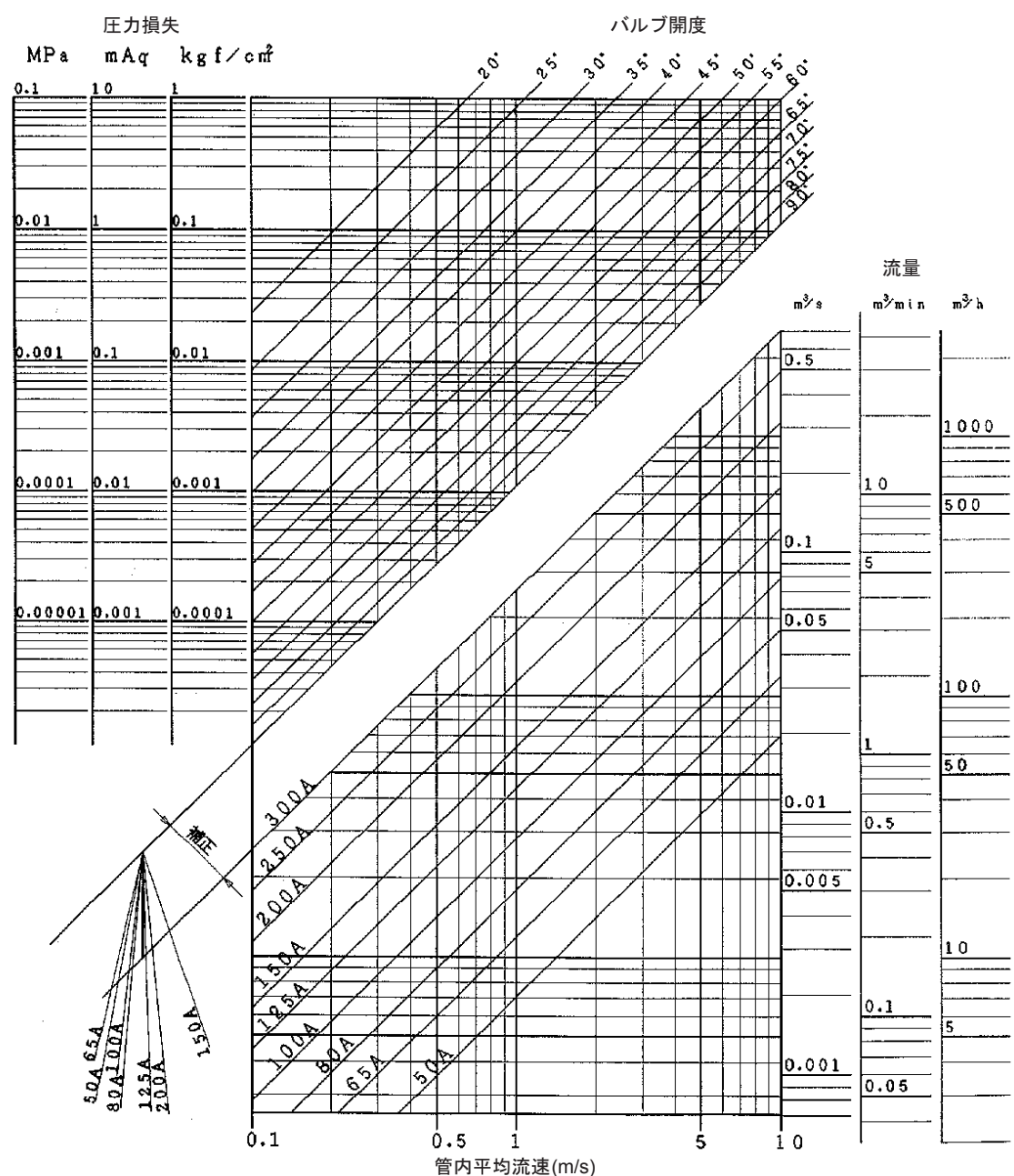
図31 形番VY6971、形番VY6978、形番VY9971バルブ接続口径選定および圧力損失線図（バルブ接続口径50～300A、流体：水）
