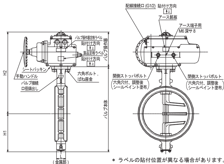
図3 形番VY6971 (スピコンなし) バルブ接続口径300Aの形状・寸法 (図の形状は全閉状態の場合)
