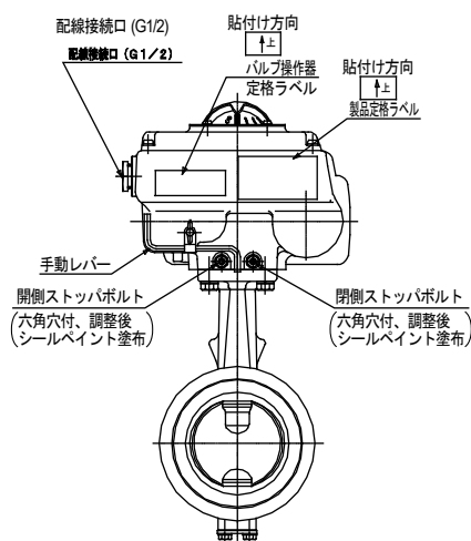
図9 形番VY6972、形番VY9972バルブ接続口径50～80Aの形状・寸法
