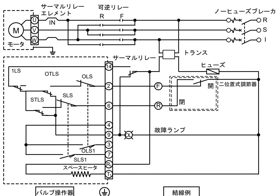
図40 LTKD-02の二位置制御式
