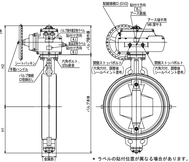
図6 形番VY6971（スピコンなし）バルブ接続口径450～500Aの形状・寸法 (図の形状はバルブ接続口径 450A、全閉状態の場合)
