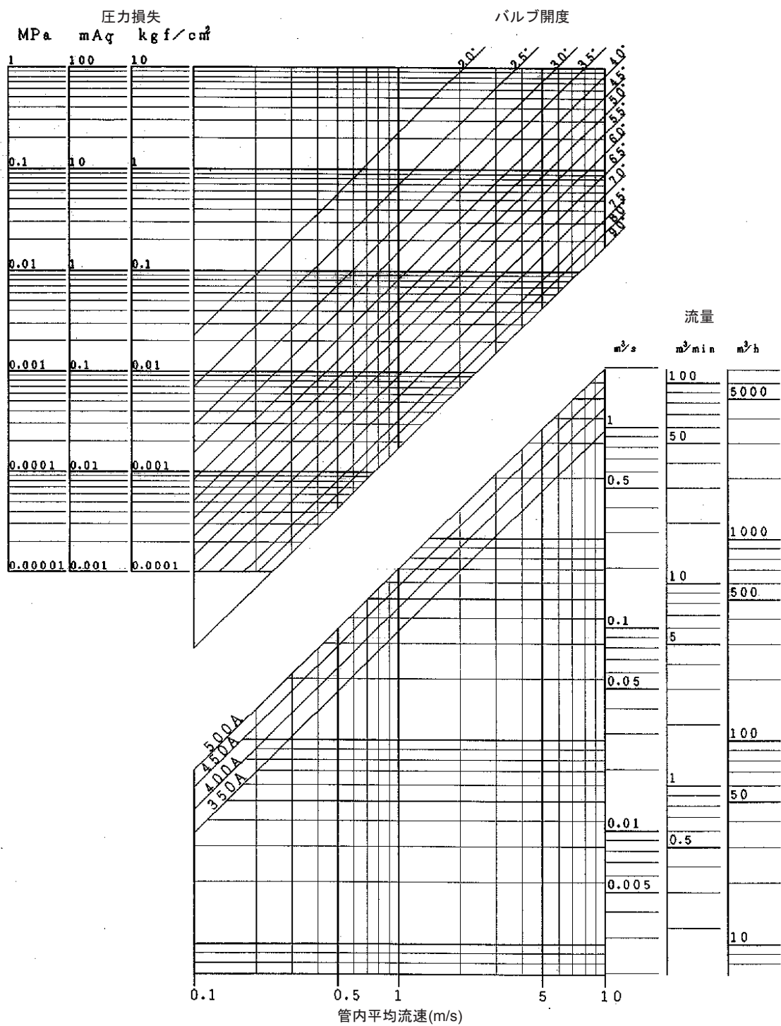
図32 形番VY6971、形番VY9971バルブ接続口径選定および圧力損失線図（バルブ接続口径350～500A、流体:水）
