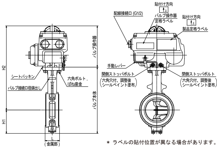
図1 形番VY6971、形番VY9971バルブ接続口径50～80Aの形状・寸法 (図の形状はバルブ接続口径 80A、全閉状態の場合)
