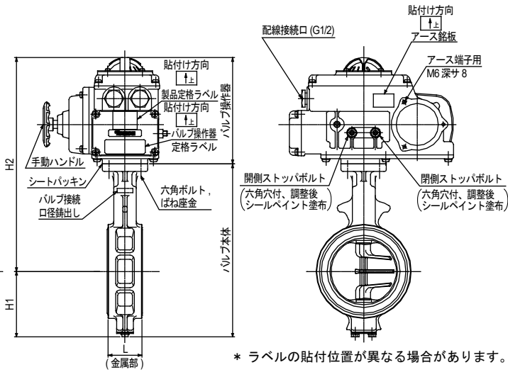
図2 形番VY6971、形番VY9971バルブ接続口径100～250Aの形状・寸法 (図の形状はバルブ接続口径 100A、全閉状態の場合)
