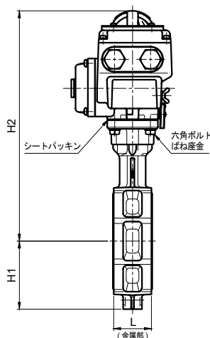
図16 形番VY6978/バルブ接続口径50～100Aの形状・寸法
