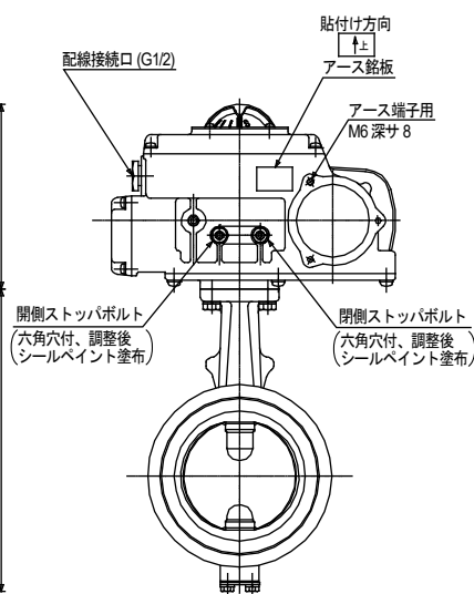
図10 形番VY6972、形番VY9972バルブ接続口径100～200Aの形状・寸法
