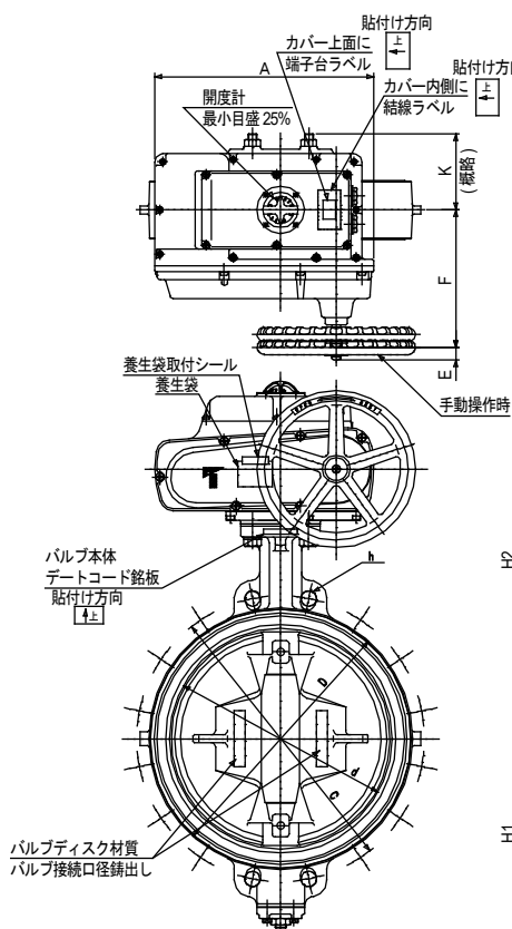
図8 形番VY6971 (スピコンあり) バルブ接続口径400~500A、形番VY9971バルブ接続口径400~500Aの形状・寸法
