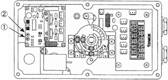
図44 開閉時間調整トリマー位置（NEL-0、1、2、2.5型）
