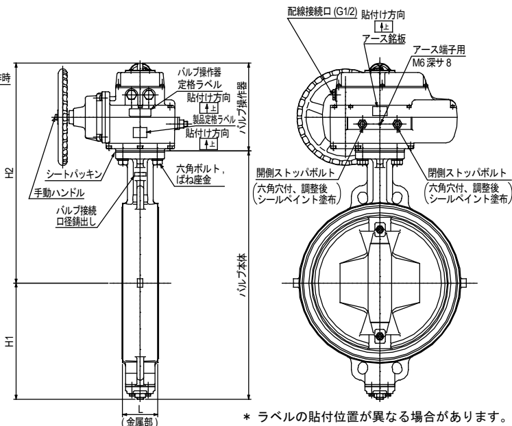
図8 形番VY6971 (スピコンあり) バルブ接続口径400~500A、形番VY9971バルブ接続口径400~500Aの形状・寸法
