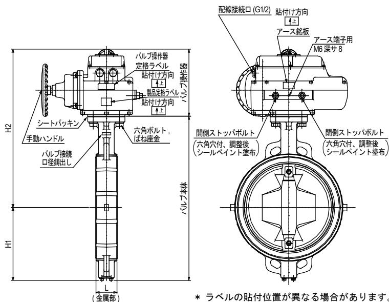
図7 形番VY6971 (スピコンあり)、形番VY9971バルブ接続口径350Aの形状・寸法
