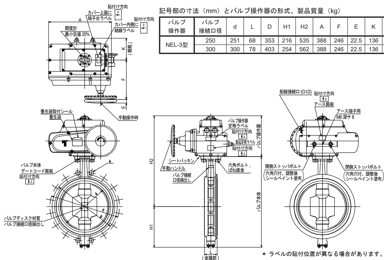
図12 形番VY6972（スピコンあり）バルブ接続口径250～300Aの形状・寸法 （図の形状はバルブ接続口径 300A、全閉状態の場合）
