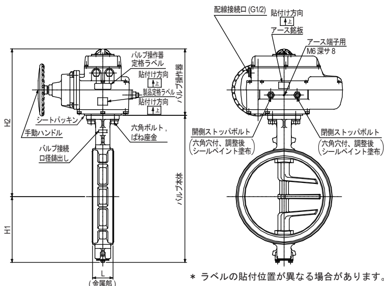
図4 形番VY6971 (スピコンあり) バルブ接続口径300Aの形状・寸法 (図の形状は全閉状態の場合)
