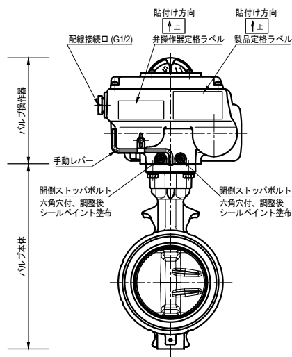
図16 形番VY6978/バルブ接続口径50～100Aの形状・寸法
