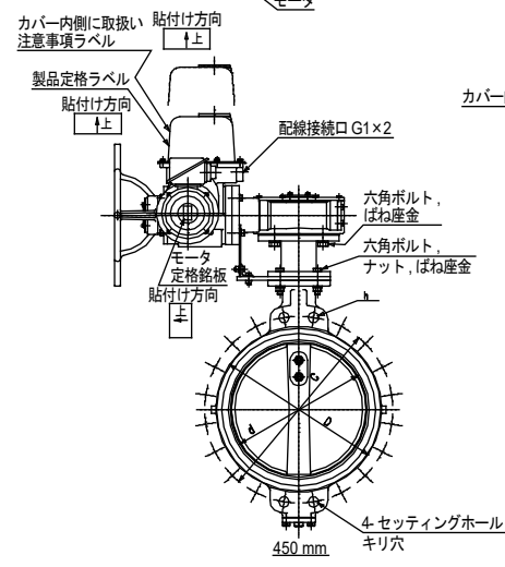
図15 形番VY6972、形番VY9972/バルブ接続口径450～500Aの形状・寸法
