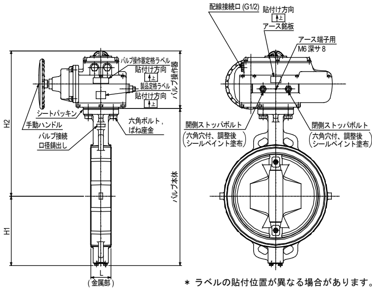
図5 形番VY6971（スピコンなし）、バルブ接続口径350～400Aの形状・寸法 (図の形状はバルブ接続口径 350A、全閉状態の場合)
