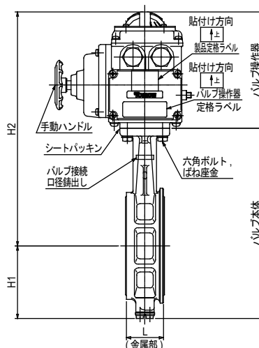
図10 形番VY6972、形番VY9972バルブ接続口径100～200Aの形状・寸法
