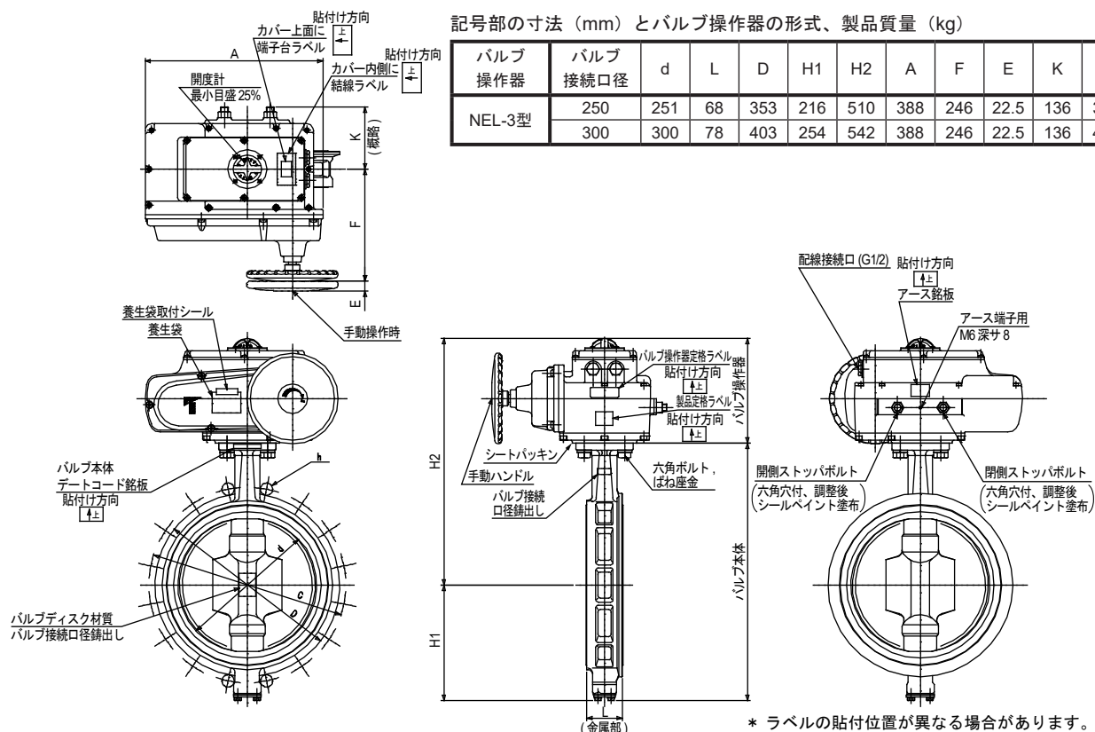
図11 形番VY6972（スピコンなし）、形番VY9972バルブ接続口径250～300Aの形状・寸法 （図の形状はバルブ接続口径 300A、全閉状態の場合）
