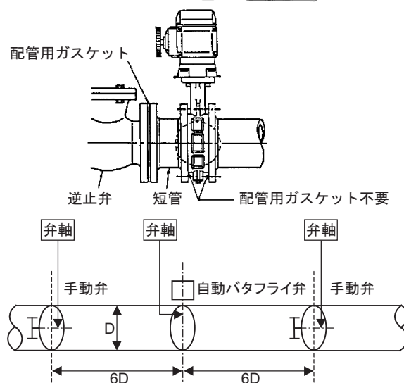
図35 取り付け上の注意
