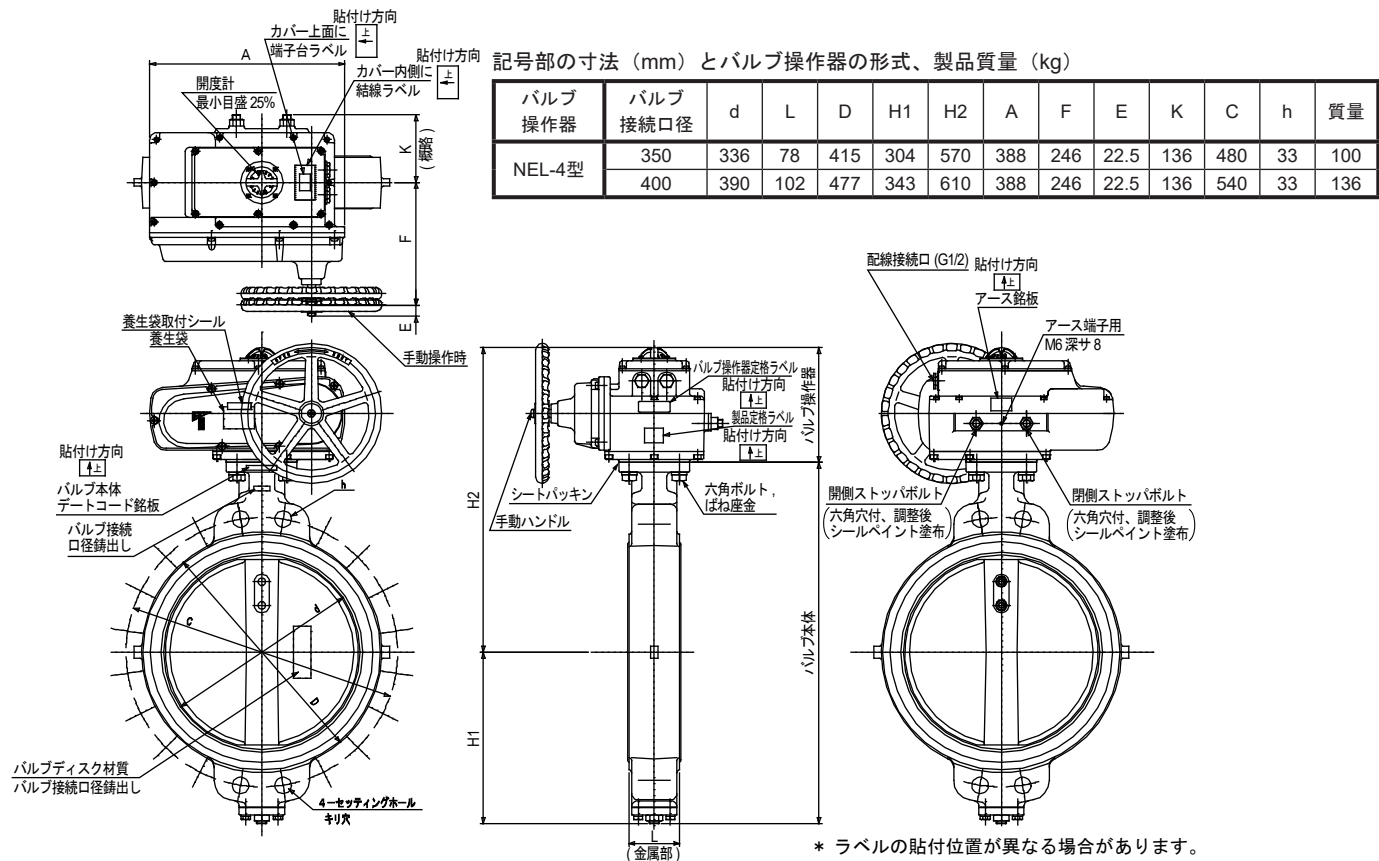
図13 形番VY6972（スピコンなし）、形番VY9972バルブ接続口径350～400Aの形状・寸法 （図の形状はバルブ接続口径 400A、全閉状態の場合）
