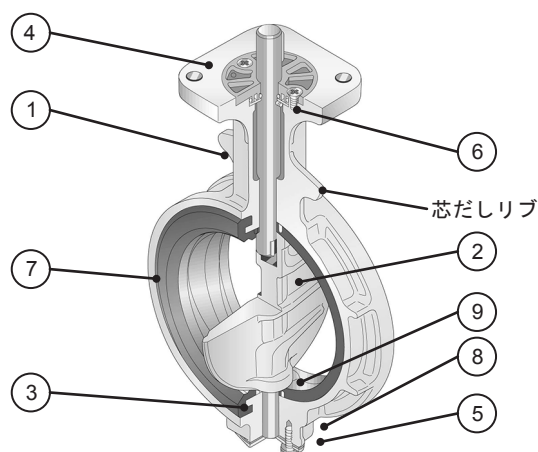
図21 形番VY6971、形番VY9971バルブ接続口径50~300Aの構造・材質
