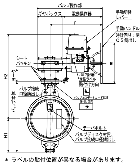
図15 形番VY6972、形番VY9972/バルブ接続口径450～500Aの形状・寸法
