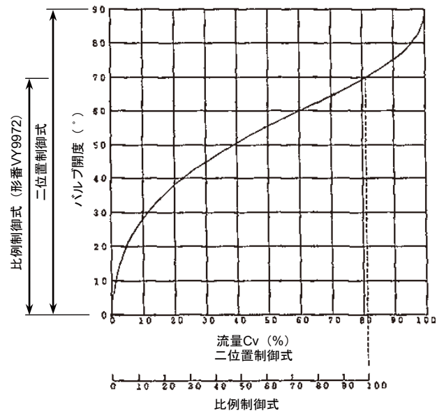
図20 形番VY9972流量特性
