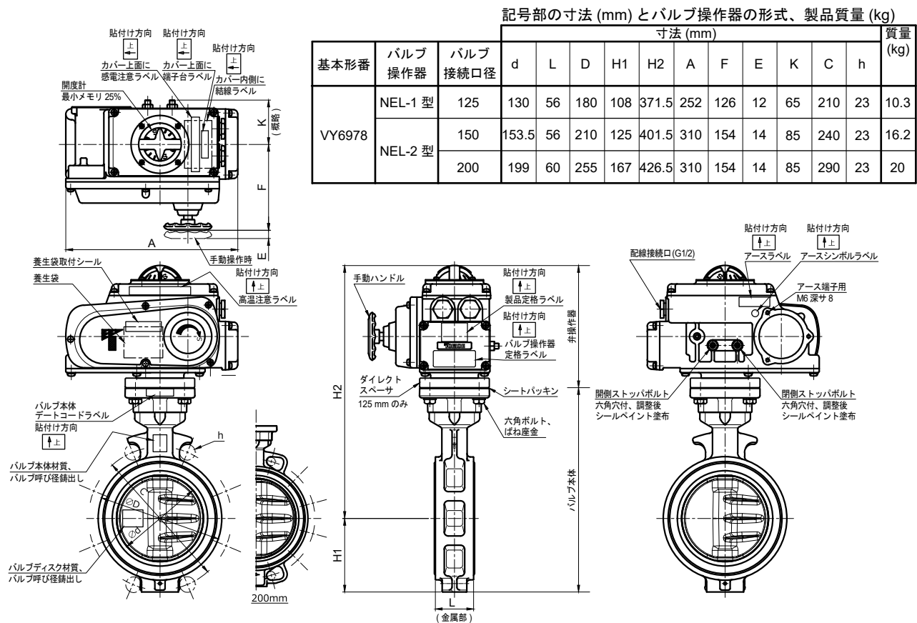
図17 形番VY6978バルブ接続口径125~200Aの形状・寸法 (図の形状はバルブ接続口径125A、全閉状態の場合)
