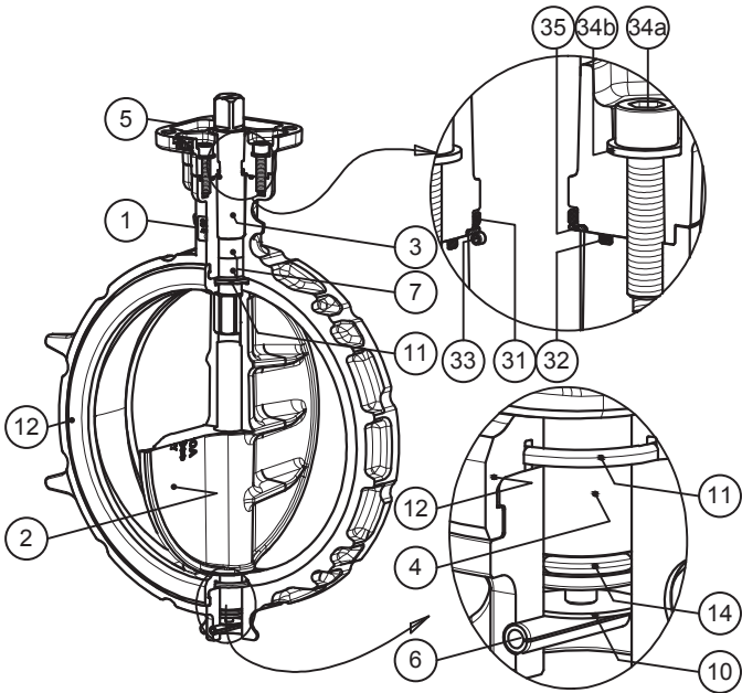
図28 形番VY6978バルブ接続口径250～300Aの構造・材質
