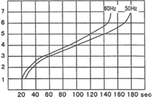
3型、4型トリマー位置と開閉時間
