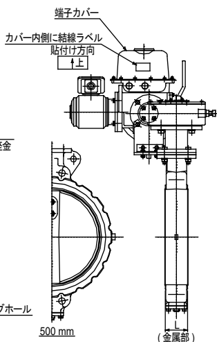
図15 形番VY6972、形番VY9972/バルブ接続口径450～500Aの形状・寸法
