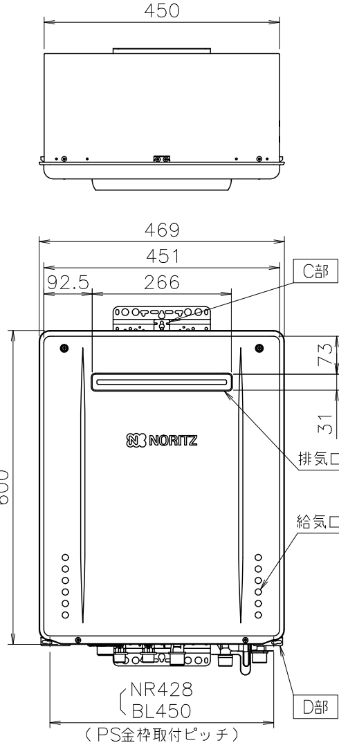
■アルコーブ取付図
