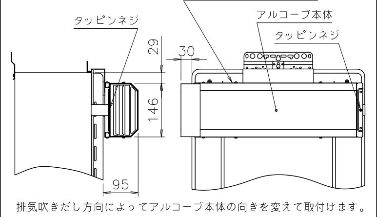
■アルコーブ取付図
