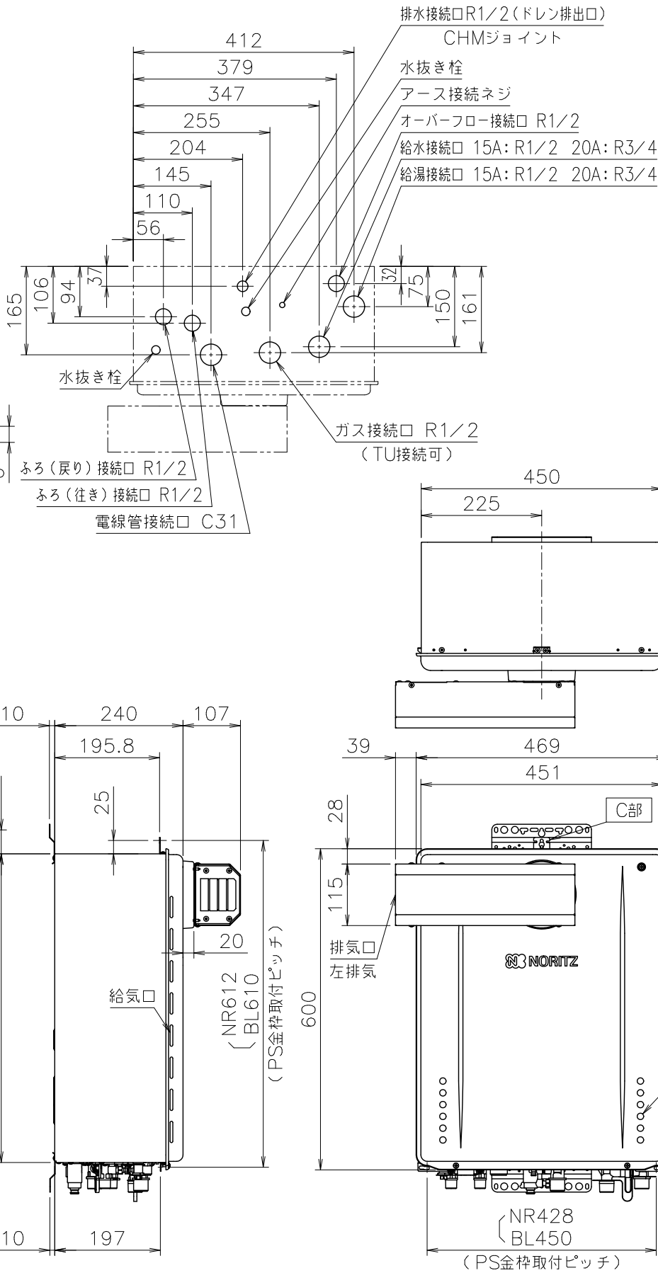
（機器上方よりの透視図）
