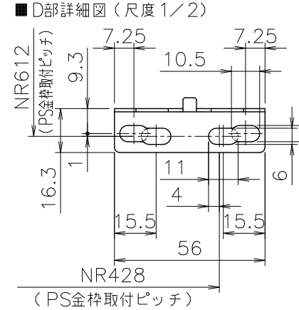
■D部詳細図(尺度1/2)
