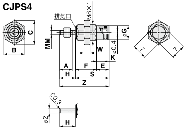
ロッド先端ねじなしの場合 CJPS4-□-B
