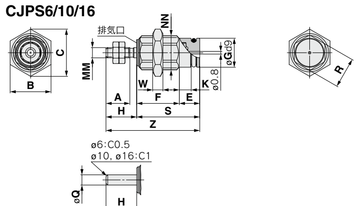
ロッド先端ねじなしの場合 CJPS□-□-B
