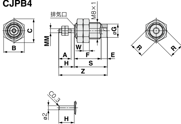
ロッド先端ねじなしの場合 CJPB4-□-B
