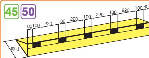
No.20B・No.25B・No.30B 寸法
