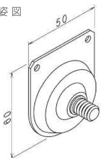
差筋D10インサートホルダー
