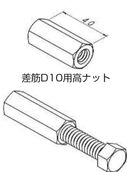
差筋D10用高ナットボルト
