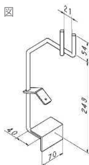
型枠養生金具 NSP45mm用
