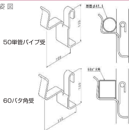
50単管 パイプ受
