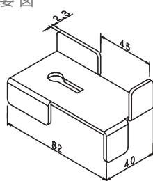
メタルジョイナー クサビ対応型45mm用
