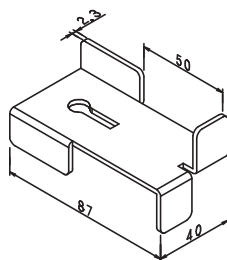
メタルジョイナー クサビ対応型50mm用
