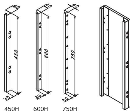
コンパネ角パイプ 姿図
