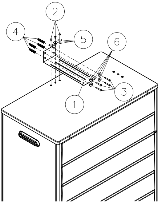
■取付要領図（概略）
