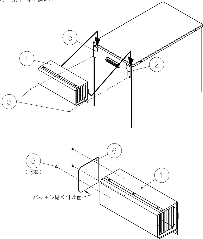
■取付完了図（概略）
